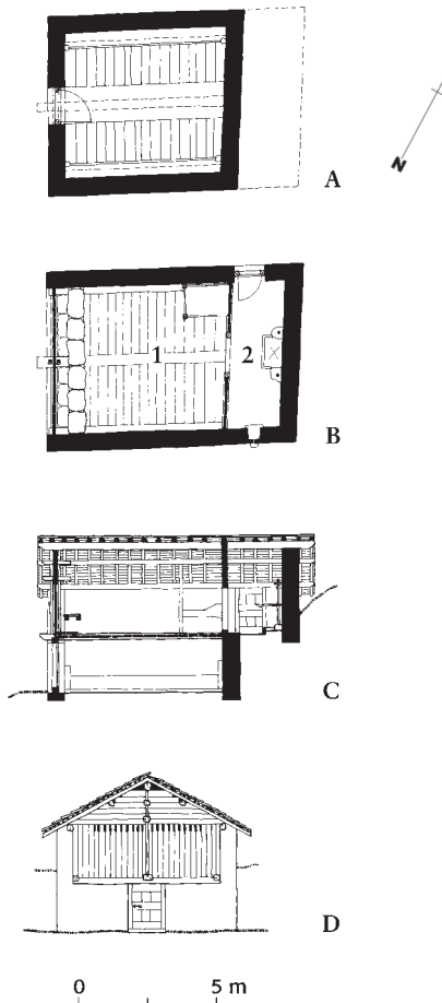
Abb. 158: Alpdörfer von Soazza. Individueller Alp-hof: A: Grundriss des Stallgeschosses; B: Grundriss des Scheunengeschosses: 1 talseitige eira mit Gebesenbank und eingebauter Bettstatt; 2 berg-seitige cassina mit Feuerstelle; C: Längsschnitt; D: Giebelfront mit Stalleingang. Mst. 1:300.
