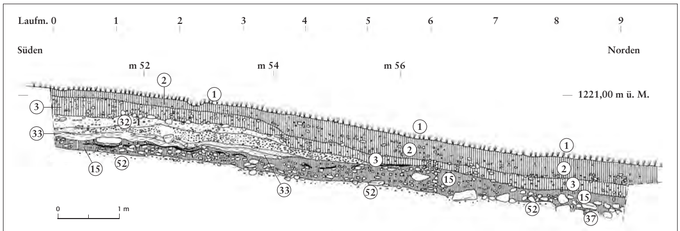
Abb. 44: Savognin, östlich Padnal. Feld 2, Westprofil (längs Kantonsstrasse). Legende: 1 Grasnarbe - 2 Humus - 3 (hell)braun, kiesig-humos - 32a grau-braun, kiesig-sandig-humos (Rüfeschutt) - 32b graue, stark kiesige Schicht (Rüfeschutt) - 33 grünliches Lehmband - 15 braun-graue, kohlig-brandige Schicht (Kulturschicht) - 52 hellbräunlich-kiesig (anstehend?). Mst. 1:60.
