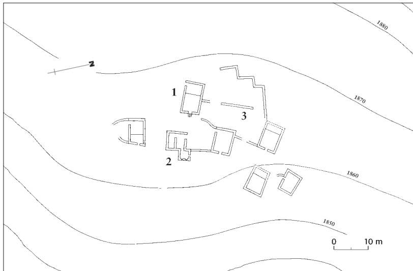
Abb. 165: Alp da Gagela. Situationsplan. Mst. 1:800.
