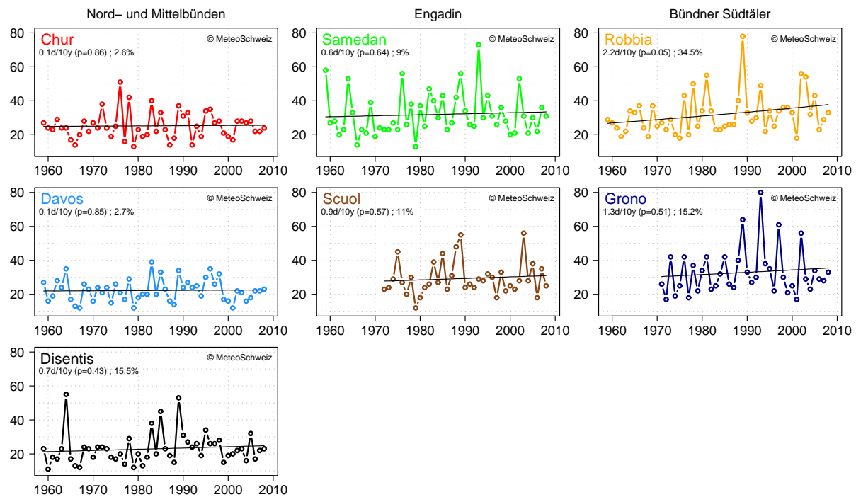
Abbildung 4.5: Zeitlicher Verlauf der maximalen Anzahl zusammenhängender Tage des Kalenderjahres für welche Tagesniederschlag <1 mm (Trockentage) für Stationen des Nord- und Mittelbündens (links, Stationen Chur, Davos, Disentis), des Engadins (mitte, Stationen Samedan und Scuol) sowie der Bündner Südtäler (rechts, Stationen Robbia und Grono). Logistische Trends in Tage / 10 Jahre sowie Signifikanzwerte und relative Abnahme über die Periode sind für jede Station angegeben.
