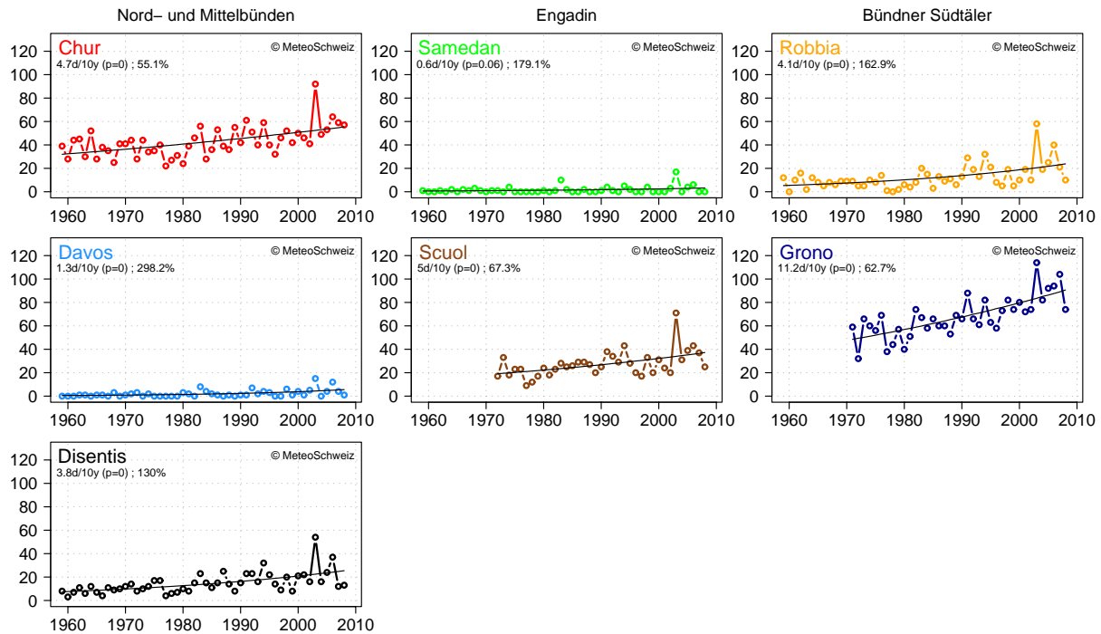
Abbildung 4.2: Zeitlicher Verlauf der Sommertage (=Anzahl Tage des Kalenderjahres mit maximaler Temperatur \geq 25^\circ\text{C} ) für Stationen des Nord- und Mittelbünden (links, Stationen Chur, Davos, Disentis), des Engadins (Mitte, Stationen Samedan und Scuol) sowie den Bündner Südtälern (rechts, Stationen Robbia und Grono). Logistische Trends in Tage / 10 Jahre sowie Signifikanzwerte und relative Abnahme über die Periode sind für jede Station angegeben.
