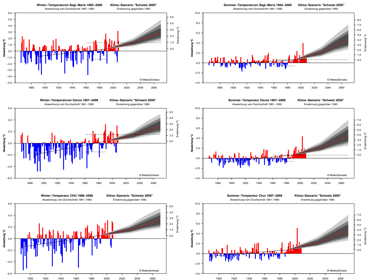
Abbildung 6.1: Langjähriger Verlauf der Wintertemperatur (Dezember bis Februar, links) und der Sommertemperatur (Juni-August, rechts) an den Messstation Segl-Maria, Davos und Chur. Der linke Bildteil zeigt die bisherige Entwicklung gemäss den Messdaten, der rechte Bildteil die erwartete zukünftige Änderung. Nähere Erläuterungen zur Grafik sind im Text zu finden.
