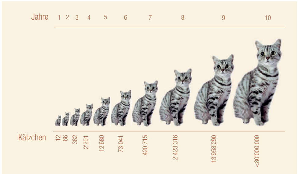
Populationsentwicklung unter idealisierten Bedingungen
