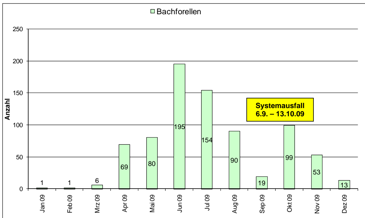
Fig.2: Monatliche Aufstiegszahlen der Bachforelle bei der Fischtreppe des KW Reichenau, Domat/Ems im Jahre 2009.
