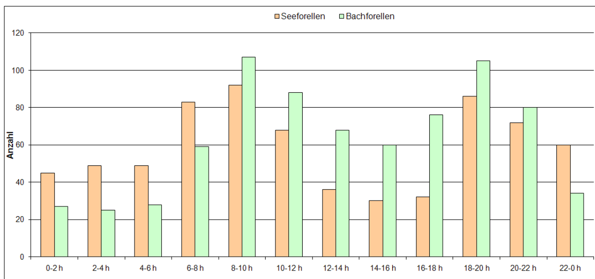
Fig.3: Tageszeitliche Aufstiegszahlen der Bach- und Bodensee-Seeforelle bei der Fischtreppe des KW Reichenau, Domat/Ems im Jahre 2009.
