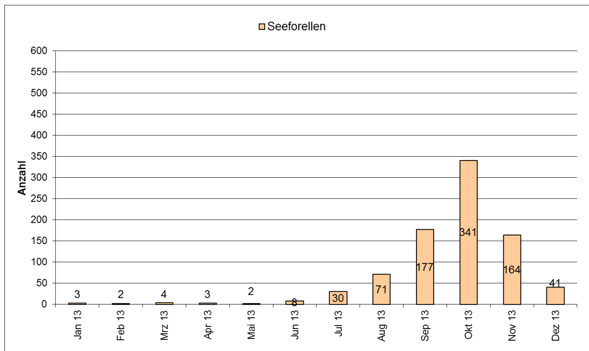
Fig.1: Monatliche Aufstiegszahlen der Bodensee-Seeforelle bei der Fischtreppe des KW Reichenau, Domat/Ems im Jahre 2013.
