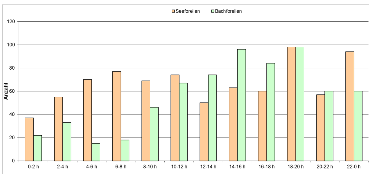
Fig.3: Tageszeitliche Aufstiegszahlen der Bach- und Bodensee-Seeforelle bei der Fischtreppe des KW Reichenau, Domat/Ems im Jahre 2013.
