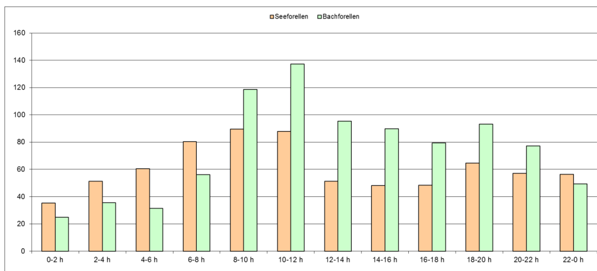
Fig.6: Tageszeitliche Aufstiegszahlen der Bach- und Bodensee-Seeforelle bei der Fisch- treppe des KW Reichenau, Domat/Ems: Langjähriges Mittel (2007-2013).
