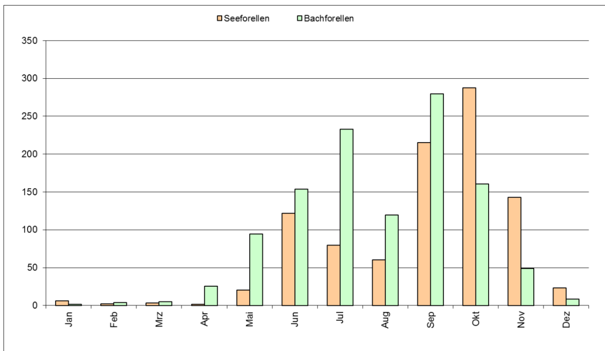
Fig.5: Monatliche Aufstiegszahlen der Bodensee-Seeforelle und Bachforellen bei der Fischtreppe des KW Reichenau, Domat/Ems: Langjähriges Mittel (2007-2013).
