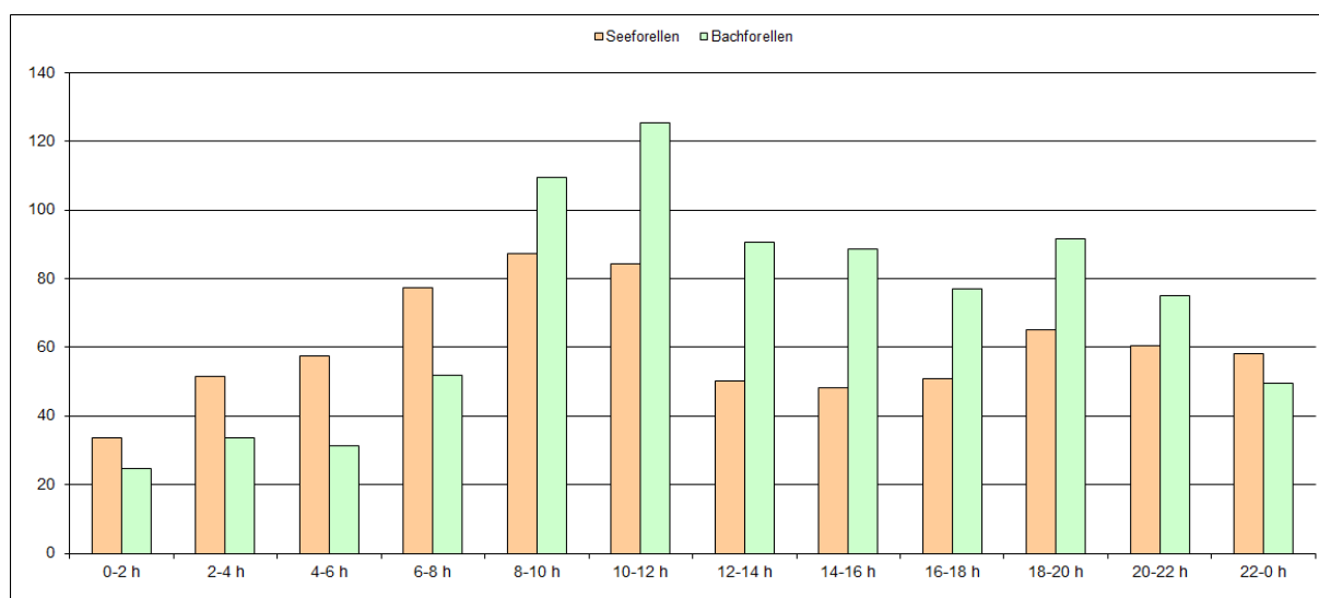
Fig.6: Tageszeitliche Aufstiegszahlen der Bach- und Bodensee-Seeforelle bei der Fisch- treppe des KW Reichenau, Domat/Ems: Langjähriges Mittel (2007-2014).
