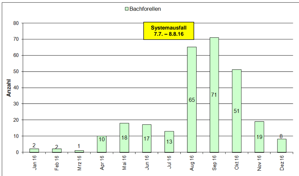
Fig.2: Monatliche Aufstiegszahlen der Bachforelle bei der Fischtreppe des KW Reichenau, Domat/Ems im Jahre 2016.
