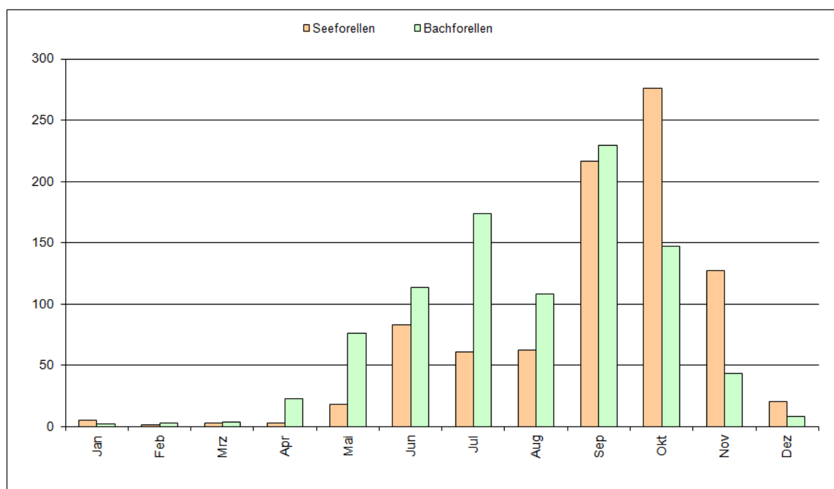
Fig.5: Monatliche Aufstiegszahlen der Bodensee-Seeforelle und Bachforellen bei der Fischtreppe des KW Reichenau, Domat/Ems: Langjähriges Mittel (2007-2016).
