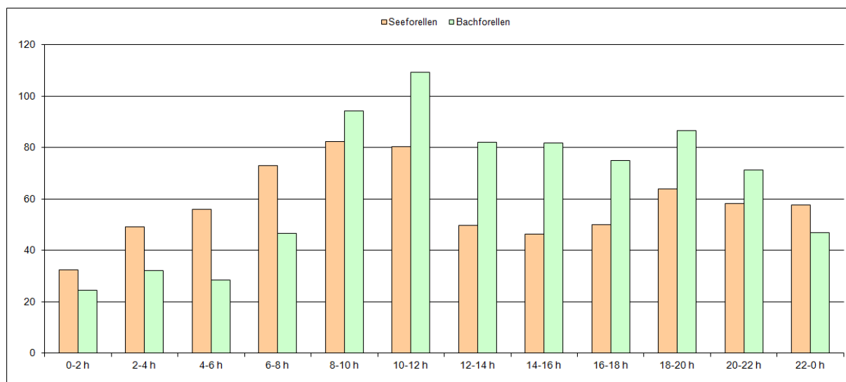
Fig.6: Tageszeitliche Aufstiegszahlen der Bach- und Bodensee-Seeforelle bei der Fisch- treppe des KW Reichenau, Domat/Ems: Langjähriges Mittel (2007-2016).
