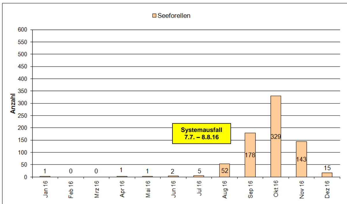
Fig.1: Monatliche Aufstiegszahlen der Bodensee-Seeforelle bei der Fischtreppe des KW Reichenau, Domat/Ems im Jahre 2016.
