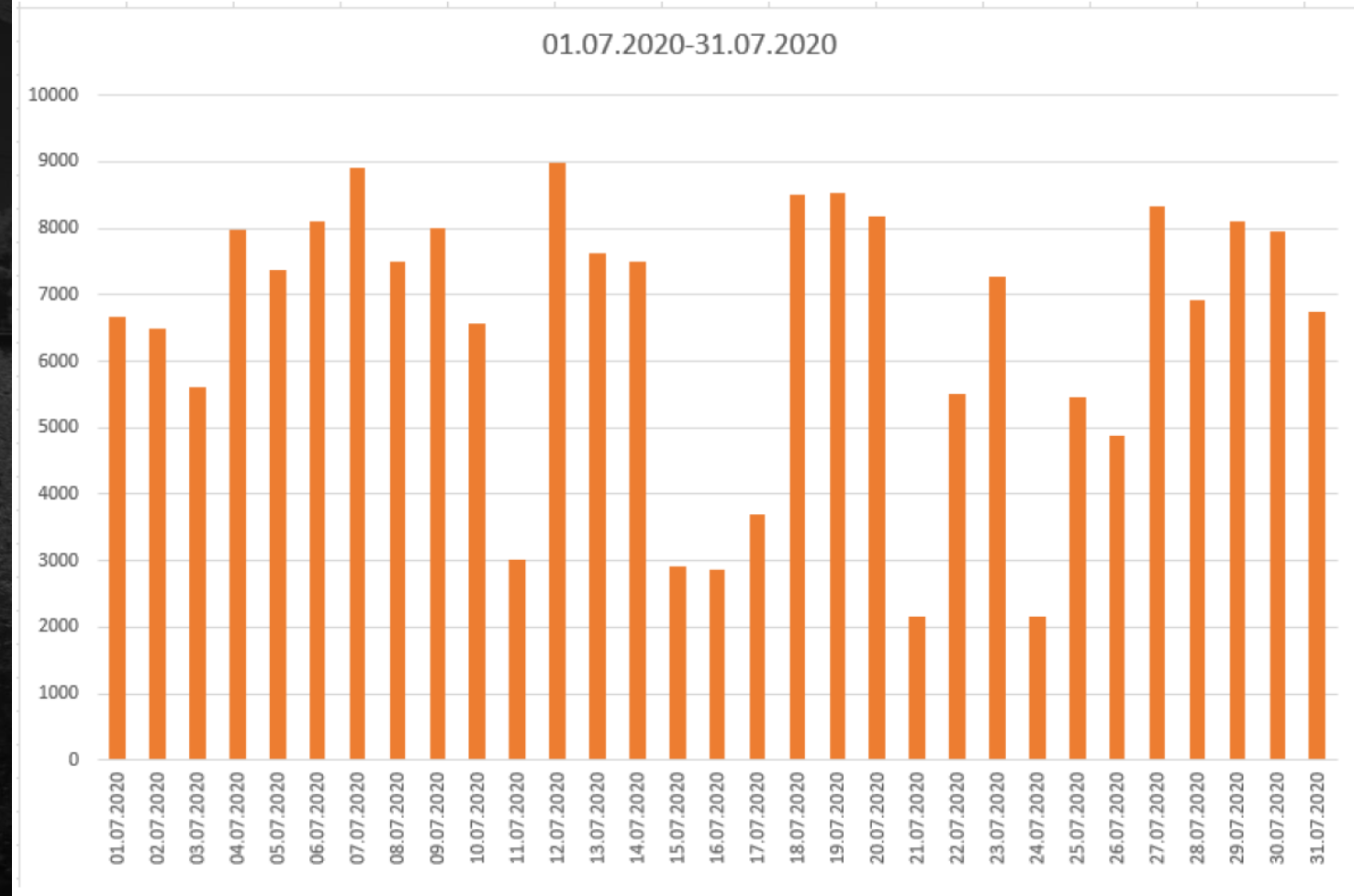
Tagesenergieproduktion in kWh von 01.07.2020 bis 31.07.2020
