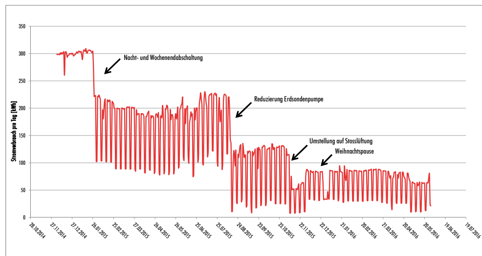
Abbildung 1: Tages-Energieverbrauch der HLK Anlage. Deutlich im Verbrauchsprofil erkennbar sind die Verbrauchsminderungen infolge der verschiedenen Massnahmen.
