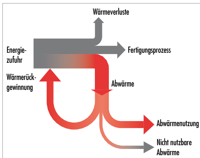
Abbildung 3: Optimierter Energiefluss.
