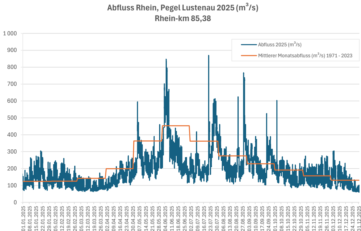
Abb. 2 Abfluss Rhein, Pegel Lustenau 2025 (m 3 /s); Rhein-km 85,38 und mittlerer Monatsabfluss Zeitreihe 1971-2023.
