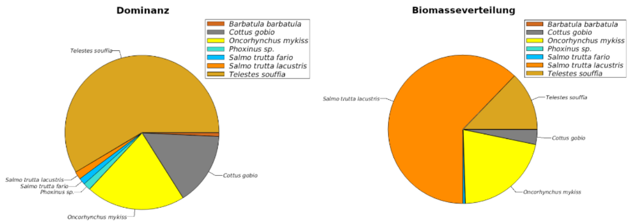
Abb. 32 Dominanzverhältnisse (links) und Biomasseverteilung (rechts) – RHE 3.
