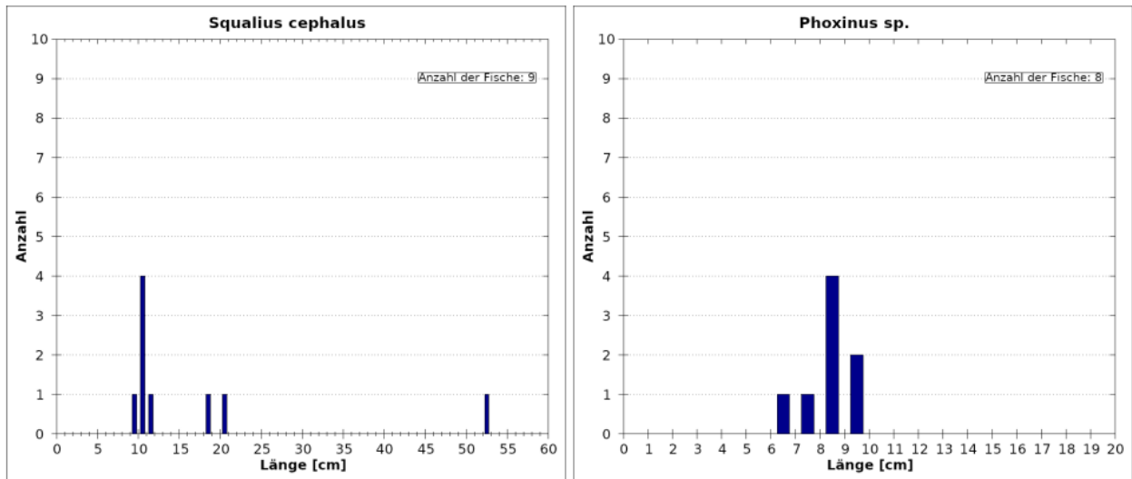
Abb. 42 Längenfrequenzdiagramm der typischen Begleitfischart Alet (links) und Elritze (rechts) – RHE 4.
