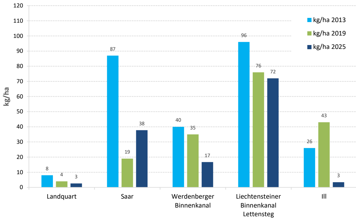
Abb. 109 Vergleich Fischbiomasse in den Zubringern – 2013, 2019 und 2025.
