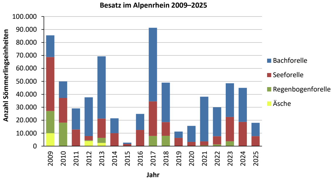
Abb. 117 Standardisierte Angaben zum Besatz im Alpenrhein der Jahre 2009–2025 in Anzahl der Sömmerringseinheiten (Hydra AG in prep).
