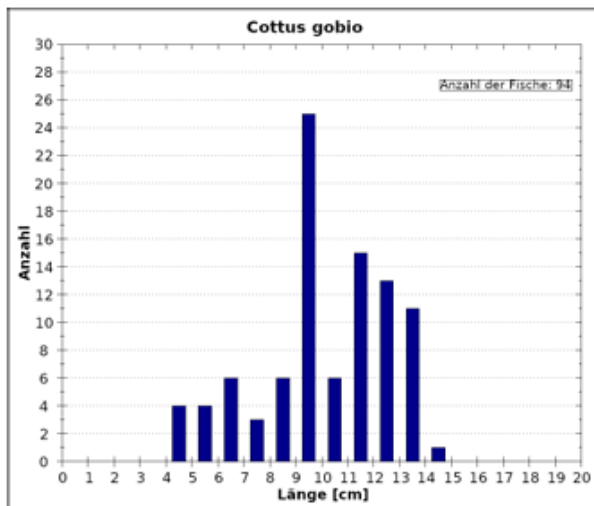
Abb. 94 Längenfrequenzdiagramm Groppe, Bewertung 1.
