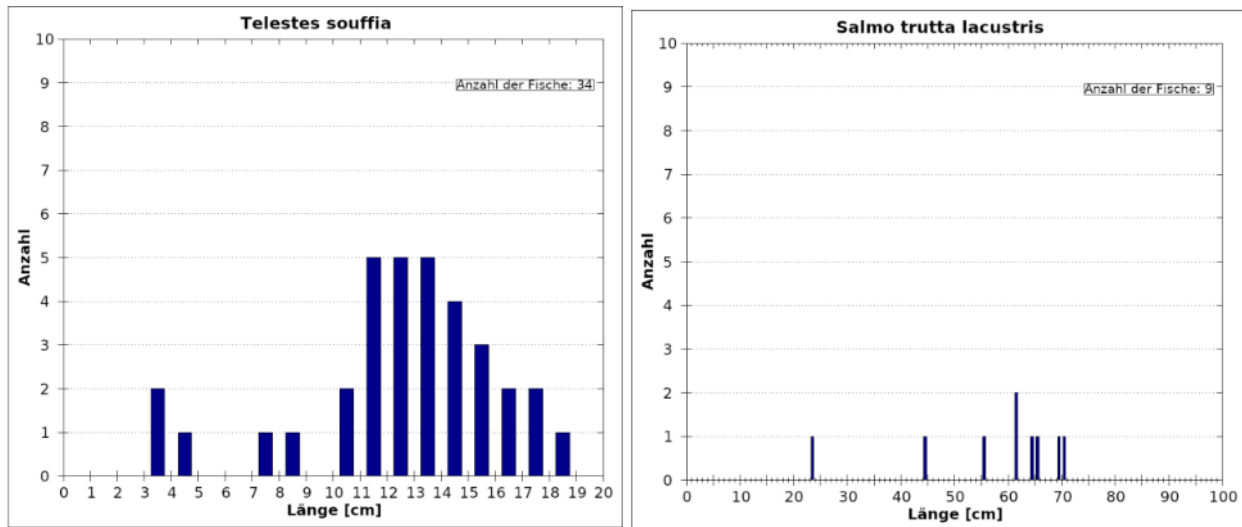
Abb. 29 Längenfrequenzdiagramm der Leitfischart Strömer (links), sowie der typischen Begleitfischart Seeforelle (rechts) – RHE 2.
