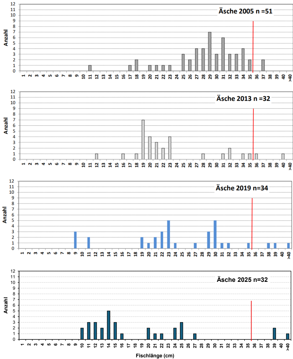
Abb. 86 Längen-Häufigkeitsverteilungen Äsche – 2005, 2013, 2019 und 2025 – Alpenrhein.
