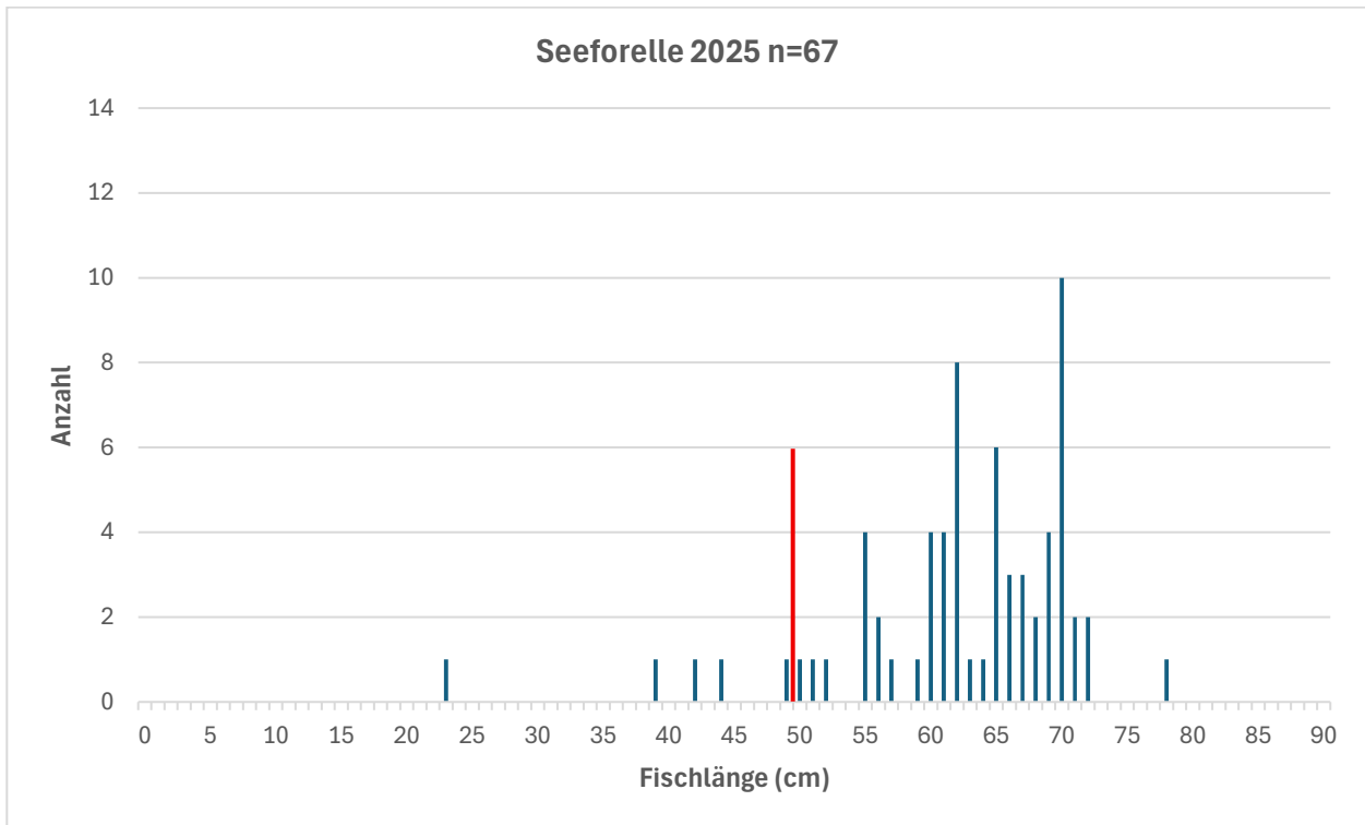
Abb. 76 Längen-Häufigkeitsverteilung Seeforelle – Alpenrhein.
