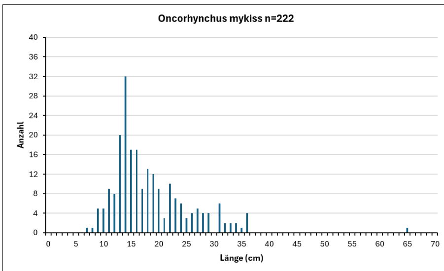
Abb. 30 Längenfrequenzdiagramm der Regenbogenforelle.
