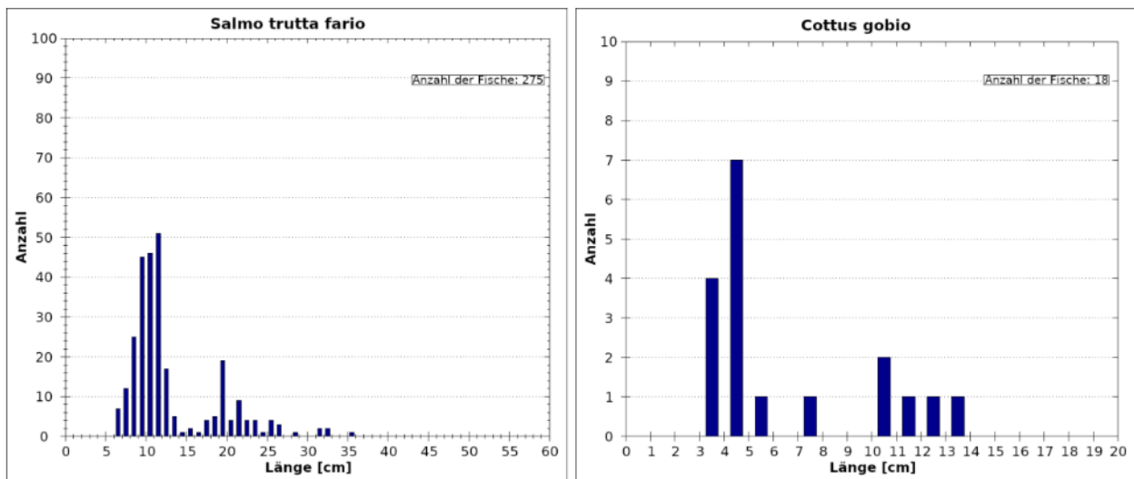
Abb. 24 Längenfrequenzdiagramm der Leitfischart Bachforelle (links) und Groppe (rechts) – RHE 1.
