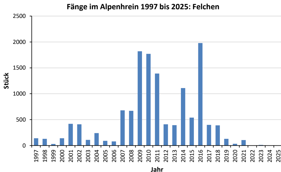
Abb. 115 Entwicklung Fangzahlen Felchen 1997 bis 2025.
