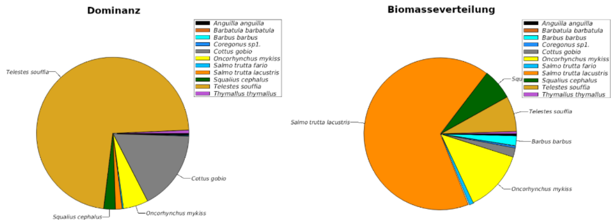
Abb. 45 Dominanzverhältnisse (links) und Biomasseverteilung (rechts) – RHE 5.
