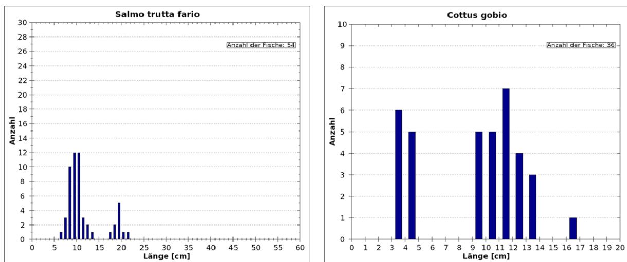
Abb. 91 Längenfrequenzdiagramm Bachforelle (links, Bewertung 3) und Längenfrequenzdiagramm Groppe (rechts, Bewertung 2)
