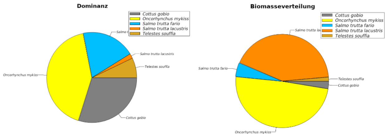
Abb. 27 Dominanzverhältnisse (links) und Biomasseverteilung (rechts) – RHE 2.
