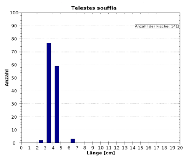
Abb. 60 Längenfrequenzdiagramm der Leitart Strömer – RHE 7.
