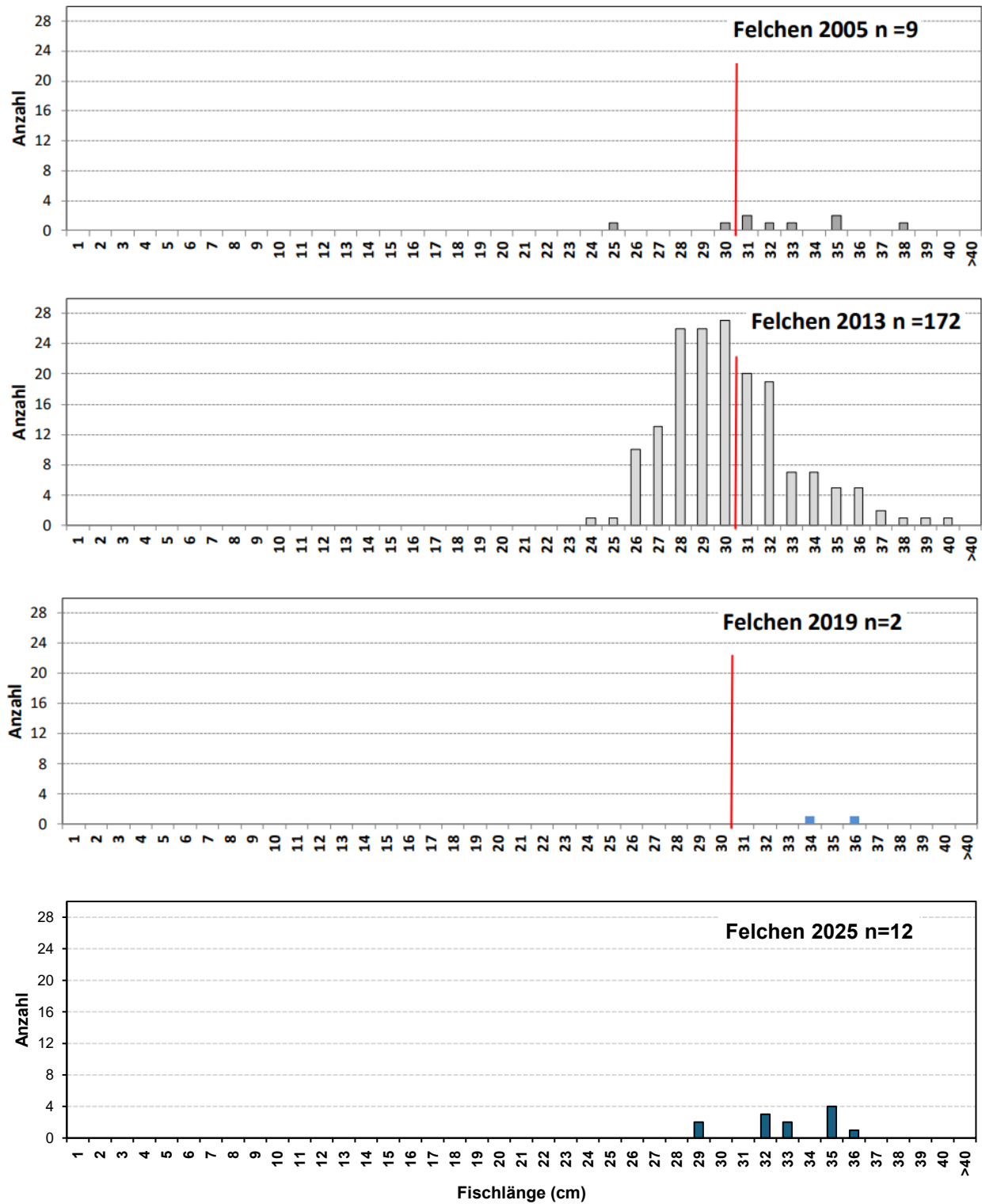
Abb. 88 Längen-Häufigkeitsverteilungen Felchen – 2005, 2013, 2019 und 2025 – Alpenrhein.
