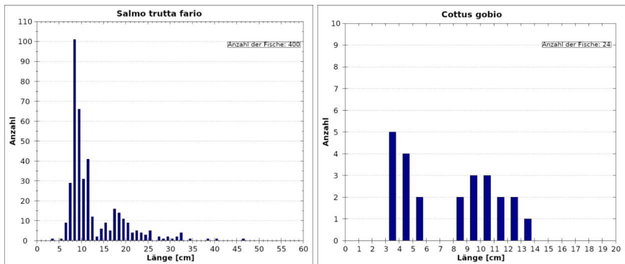
Abb. 19 Populationsstruktur der Leitfischarten Bachforelle (links) und Groppe (rechts) – Hinterrhein.
