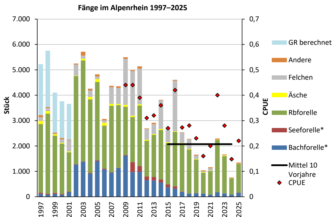
Abb. 110 Fangstatistik Alpenrhein 1997 bis 2025, aus Jahresbericht der Fischereifachstellen 2025 (Hydra AG in prep.).
