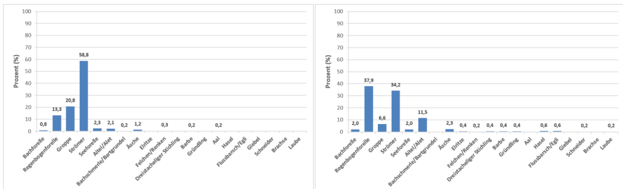
Abb. 66 Artenverteilung RHE 5 (links) und RHE 6 (rechts) – Alpenrhein.
