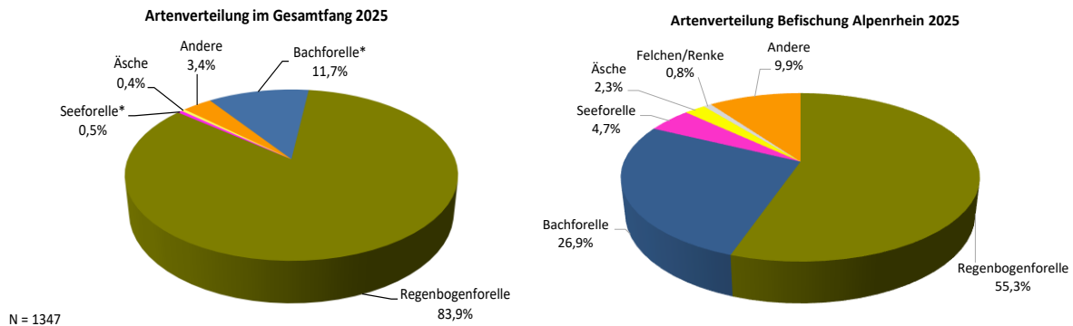
Abb. 111 Artenverteilung für den gesamten Alpenrhein anhand der Fangstatistik 2025 (links; Hydra AG in prep.); sowie anhand der Befischungsergebnisse 2025 (ohne Kleinfischarten).
