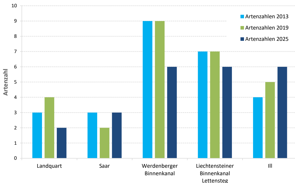
Abb. 107 Vergleich der Artenzahlen in den Zubringern, 2013, 2019 und 2025.
