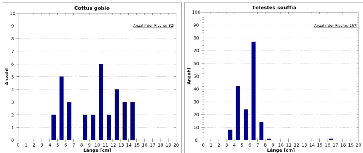
Abb. 54 Längenfrequenzdiagramm der Leitart Groppe (links) und Strömer (rechts) – RHE 6.
