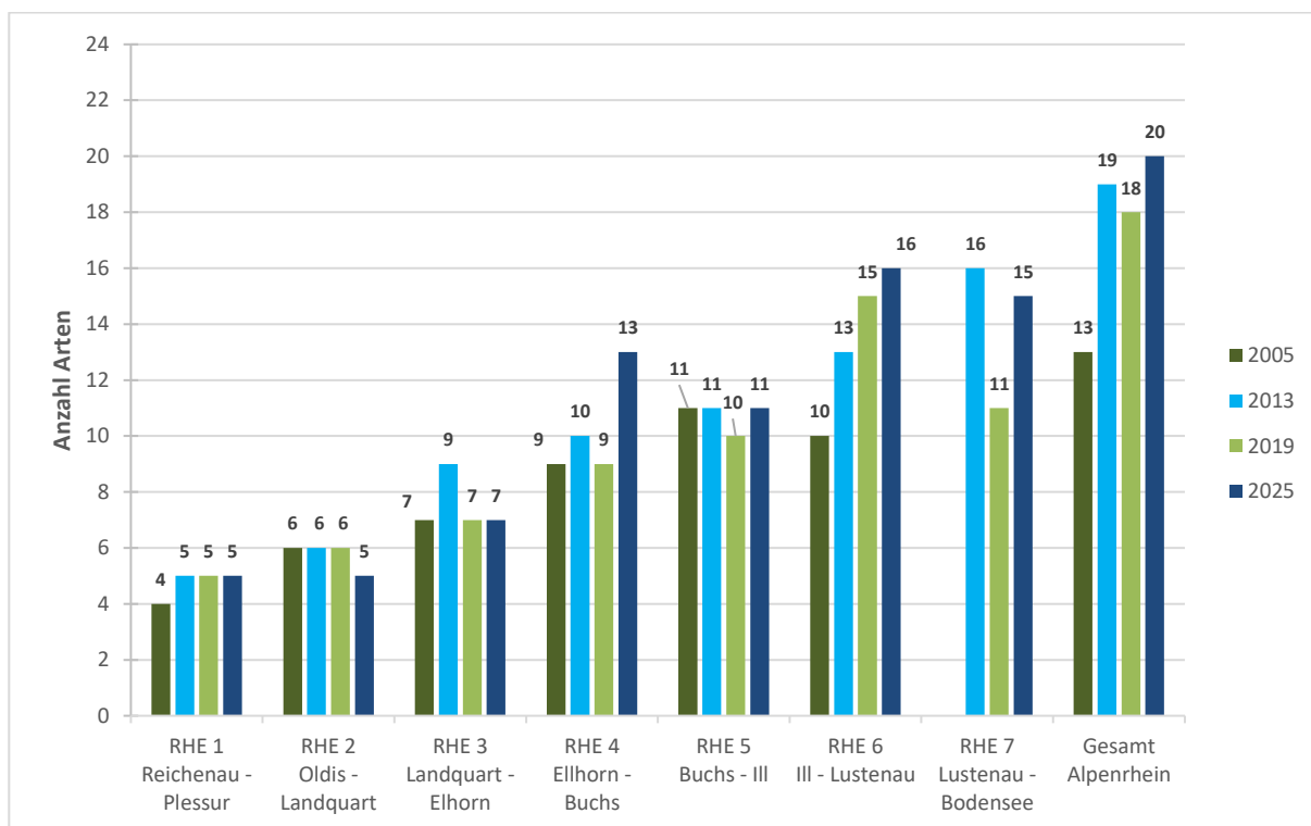
Abb. 78 Vergleich Gesamtartenzahl 2005 (ohne RHE 7), 2013, 2019 und 2025.
