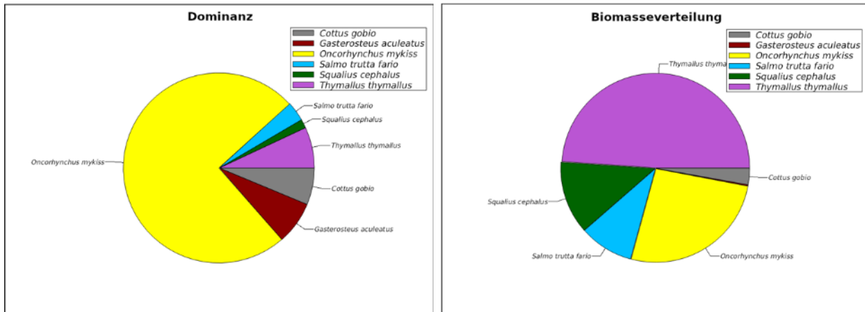
Abb. 101 Dominanz und Biomasseverteilung Liechtensteiner Binnenkanal – Lettensteg.
