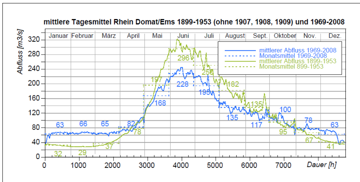
Abb. 7 Mittlere Tagesabflüsse und Monatsmittel im Rhein bei Domat/Ems für die Perioden von 1899 bis und mit 1953 (ohne 1907 bis 1909) und von 1969 bis und mit 2008 (Datenbasis Tagesmittelwerte; Ziffern: Monatsmittel) (Zarn, 2012, Frangez et al., 2020)
