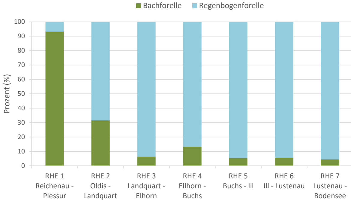
Abb. 68 Dominanzverhältnis Bach- und Regenbogenforelle im Längsverlauf – Alpenrhein.
