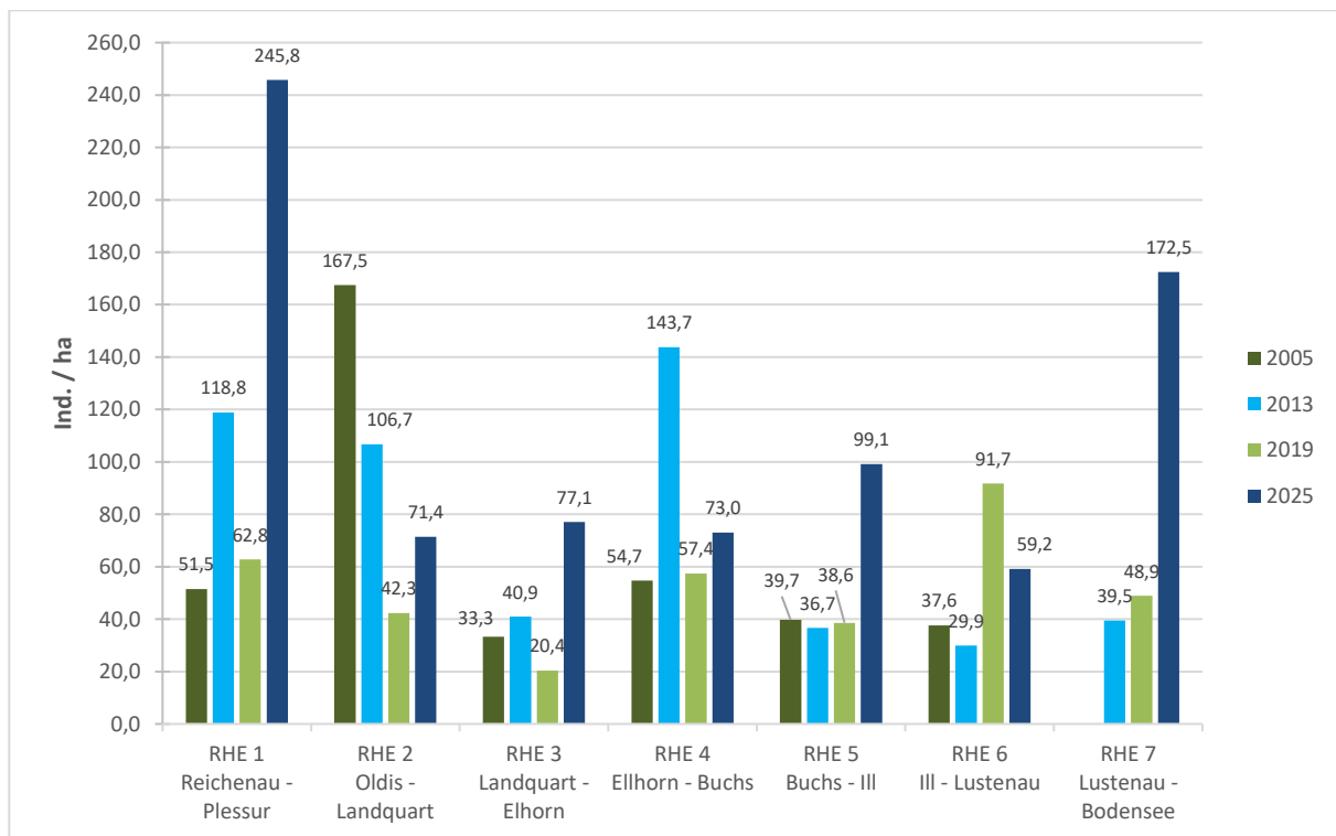
Abb. 80 Vergleich Individuendichten pro Abschnitt 2005, 2013, 2019 und 2025 – Alpenrhein
