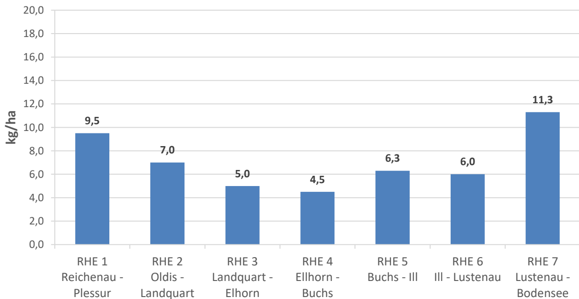
Abb. 70 Biomassen (kg/ha) innerhalb der Untersuchungsabschnitte 2025.
