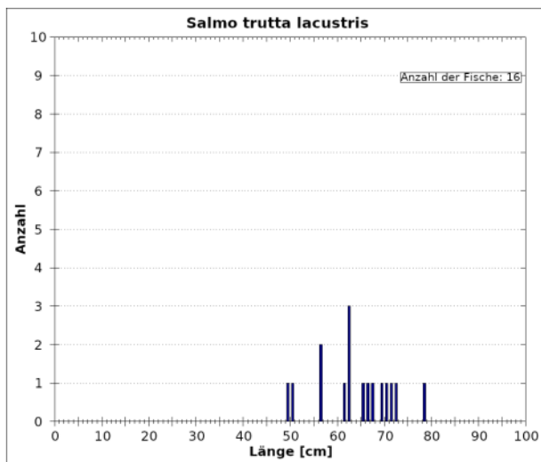
Abb. 43 Längenfrequenzdiagramm der typischen Begleitfischart Seeforelle – RHE 4.
