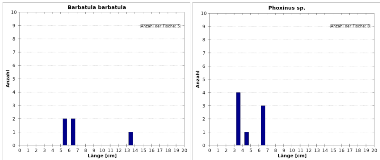
Abb. 36 Längenfrequenzdiagramm der typischen Begleitfischart Bartgrundel (links) und Elritze (rechts) – RHE 3.
