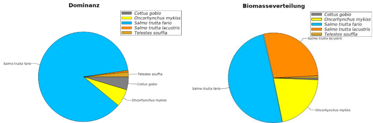
Abb. 20 Dominanzverhältnisse (links) und Biomasseverteilung (rechts) – RHE 1.
