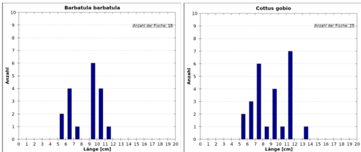
Abb. 98 Längenfrequenzdiagramm der Leitarten Bachschmerle (links) und Groppe (rechts), jeweils mit der Bewertung 2.
