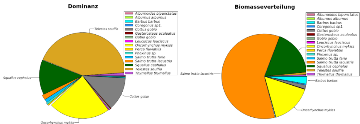
Abb. 51 Dominanzverhältnisse (links) und Biomasseverteilung (rechts) – RHE 6.
