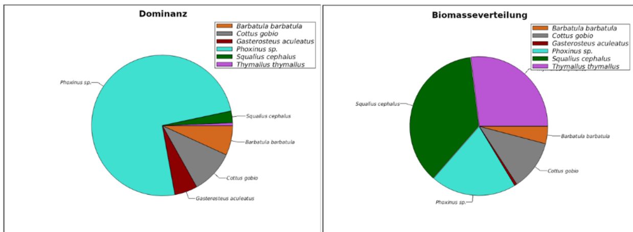
Abb. 97 Dominanz und Biomasseverteilung Werdenberger Binnenkanal.
