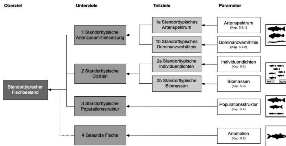
Abb. 13 Zielhierarchie mit Parametern zur Bewertung der Ziele (Achermann et al., 2024).
