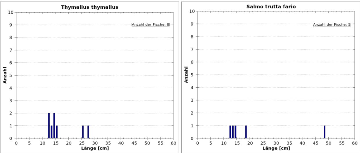
Abb. 46 Längenfrequenzdiagramm der Leitart Äsche (links) und Bachforelle (rechts) – RHE 5.
