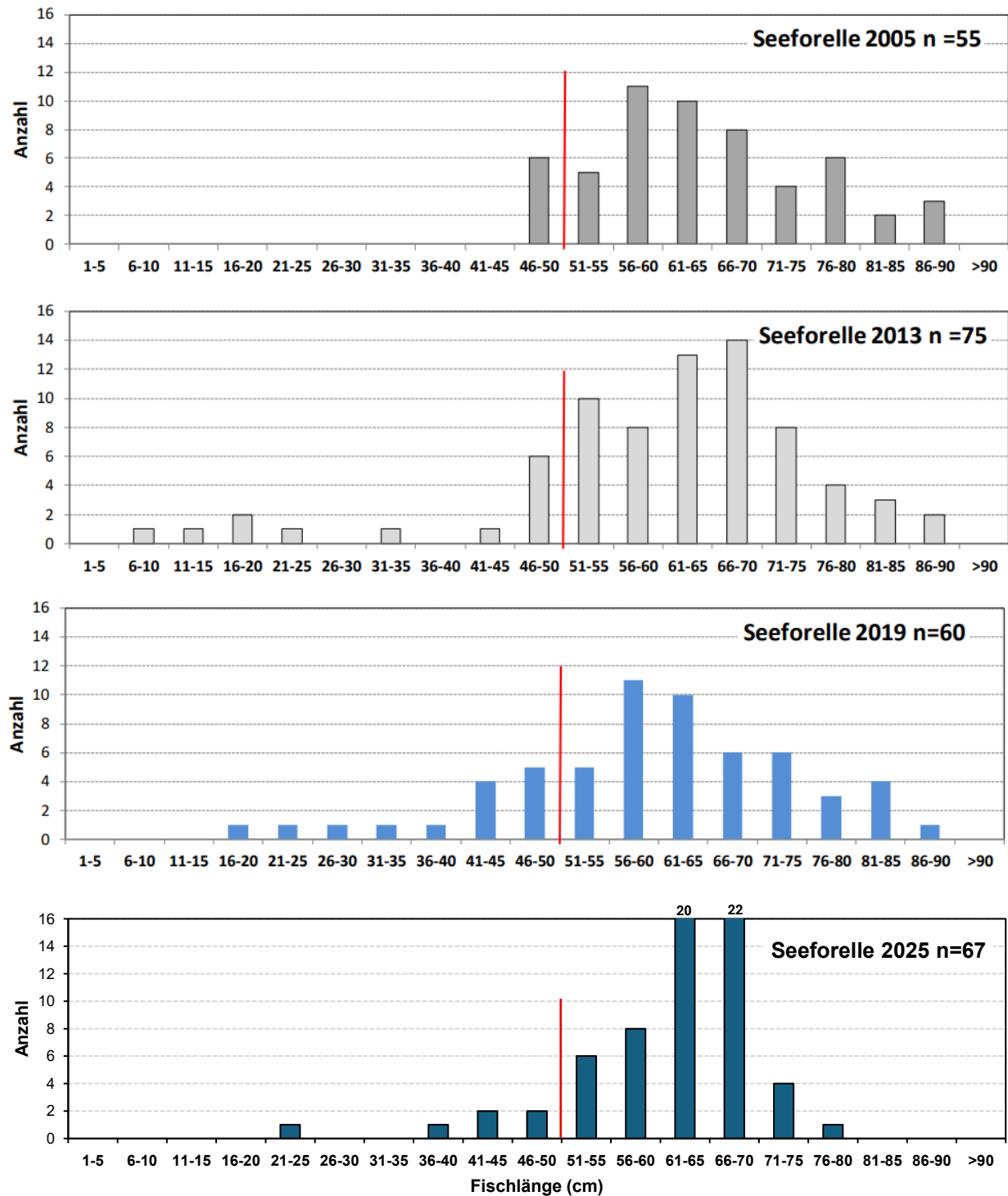
Abb. 87 Längen-Häufigkeitsverteilungen Seeforelle – 2005, 2013, 2019 und 2025 – Alpenrhein.
