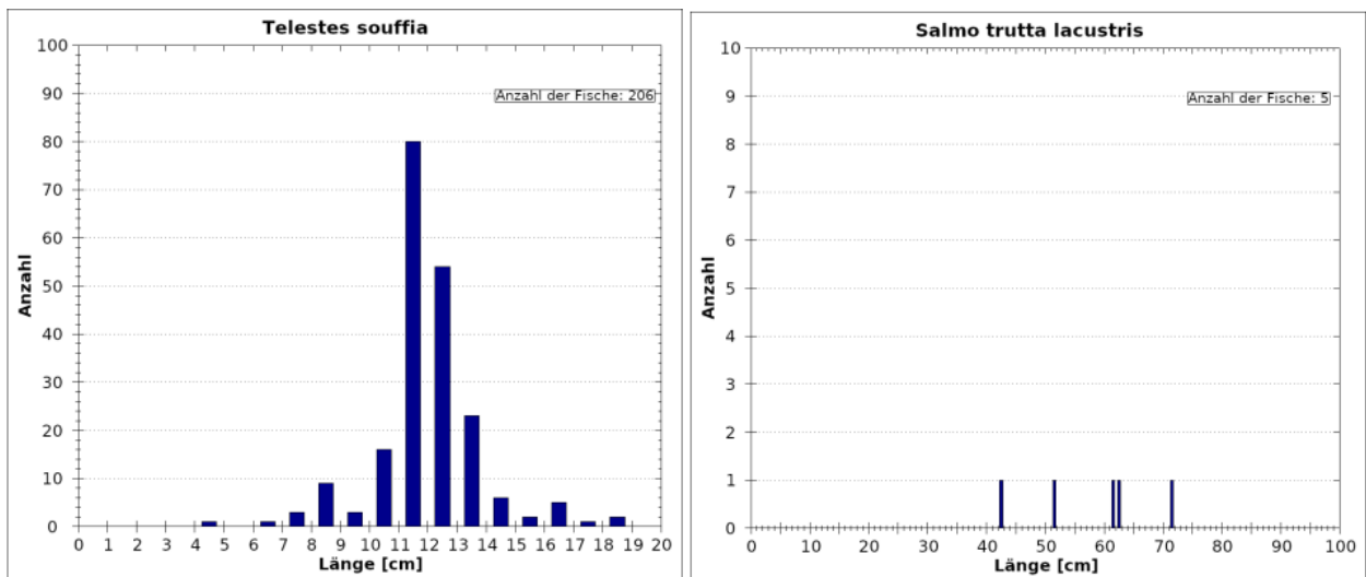
Abb. 35 Längenfrequenzdiagramm der Leitfischart Strömer (links), sowie der typischen Begleitfischart Seeforelle (rechts) – RHE 3.
