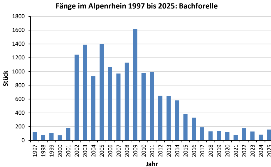
Abb. 113 Entwicklung Fangzahlen Bachforelle 1997 bis 2025.
