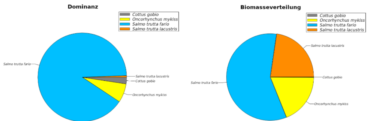
Abb. 15 Dominanzverhältnisse (links) und Biomasseverteilung (rechts) – Vorderrhein.
