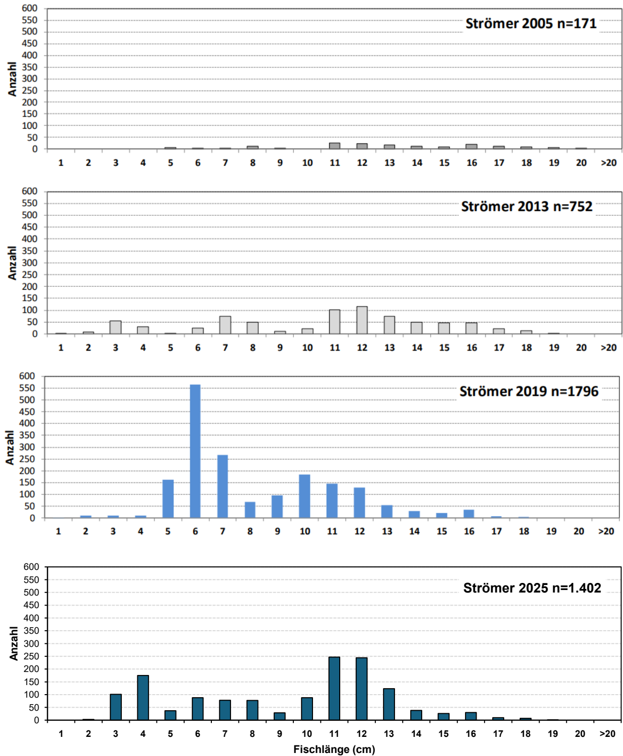
Abb. 84 Längen-Häufigkeitsverteilungen Strömer – 2005, 2013, 2019 und 2025 – Alpenrhein.
