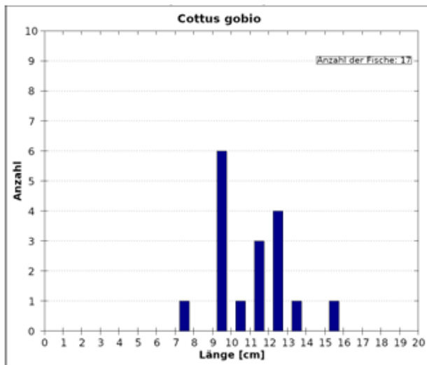
Abb. 103 Längenfrequenzdiagramm Koppe, Bewertung 3.
