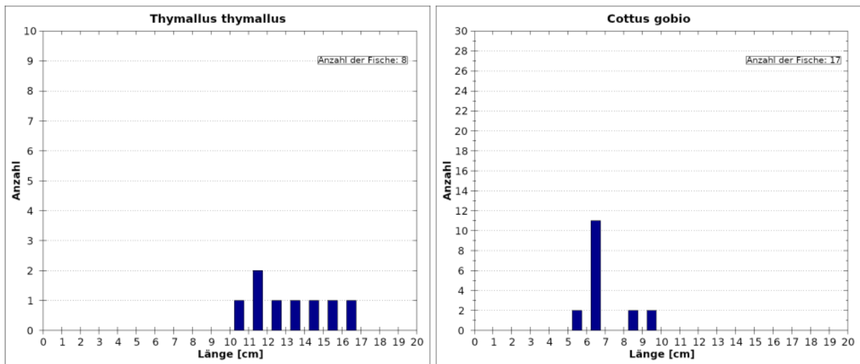
Abb. 59 Längenfrequenzdiagramm der Leitart Äsche (links) und Groppe (rechts) – RHE 7.
