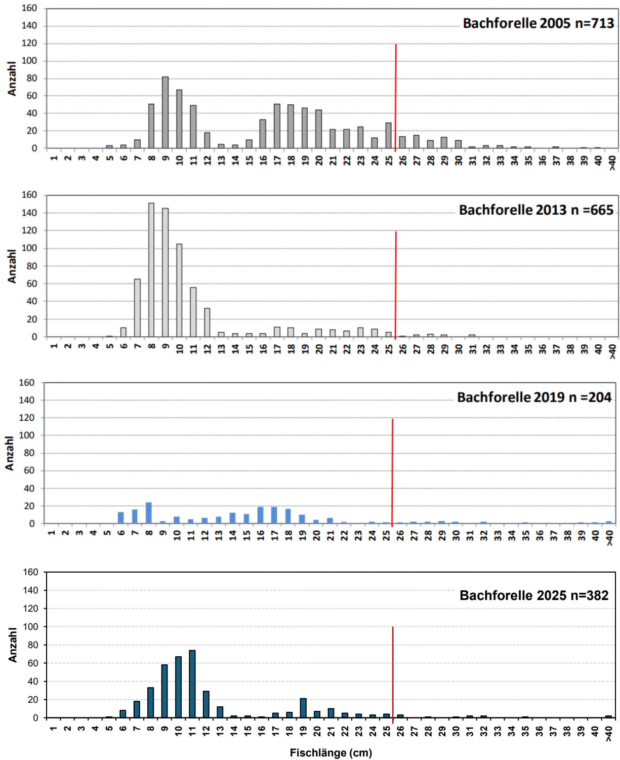
Abb. 82 Längen-Häufigkeitsverteilungen Bachforelle – 2005, 2013, 2019 und 2025 – Alpenrhein.
