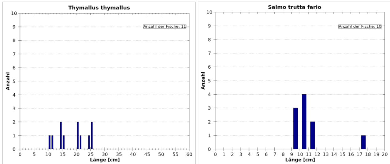
Abb. 53 Längenfrequenzdiagramm der Leitart Äsche (links) und Bachforelle (rechts) – RHE 6.
