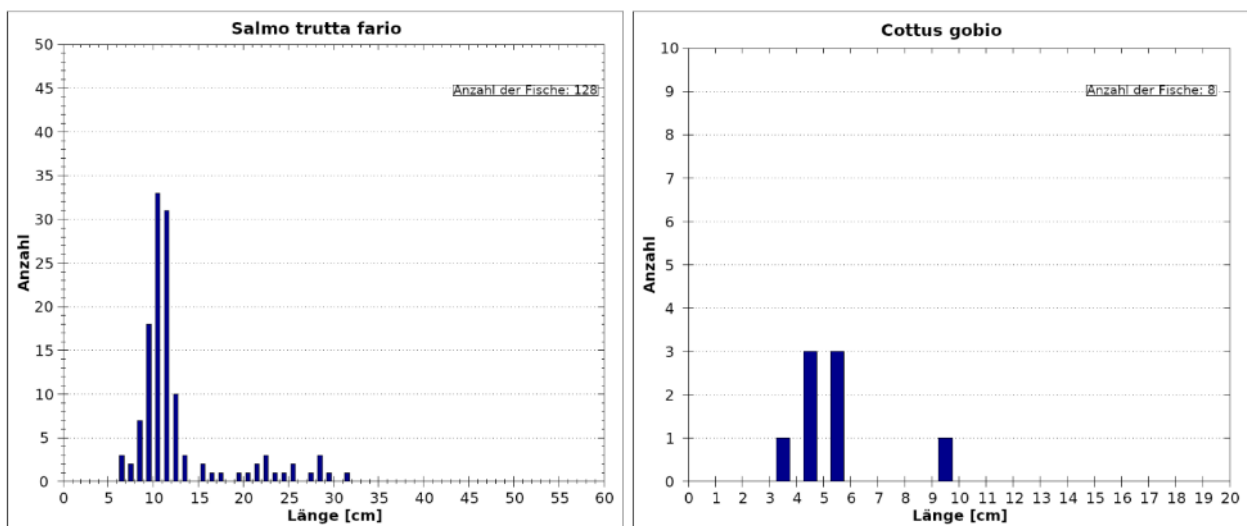
Abb. 16 Populationsstruktur der Leitfischarten Bachforelle (links) und Groppe (rechts) – Vorderrhein.
