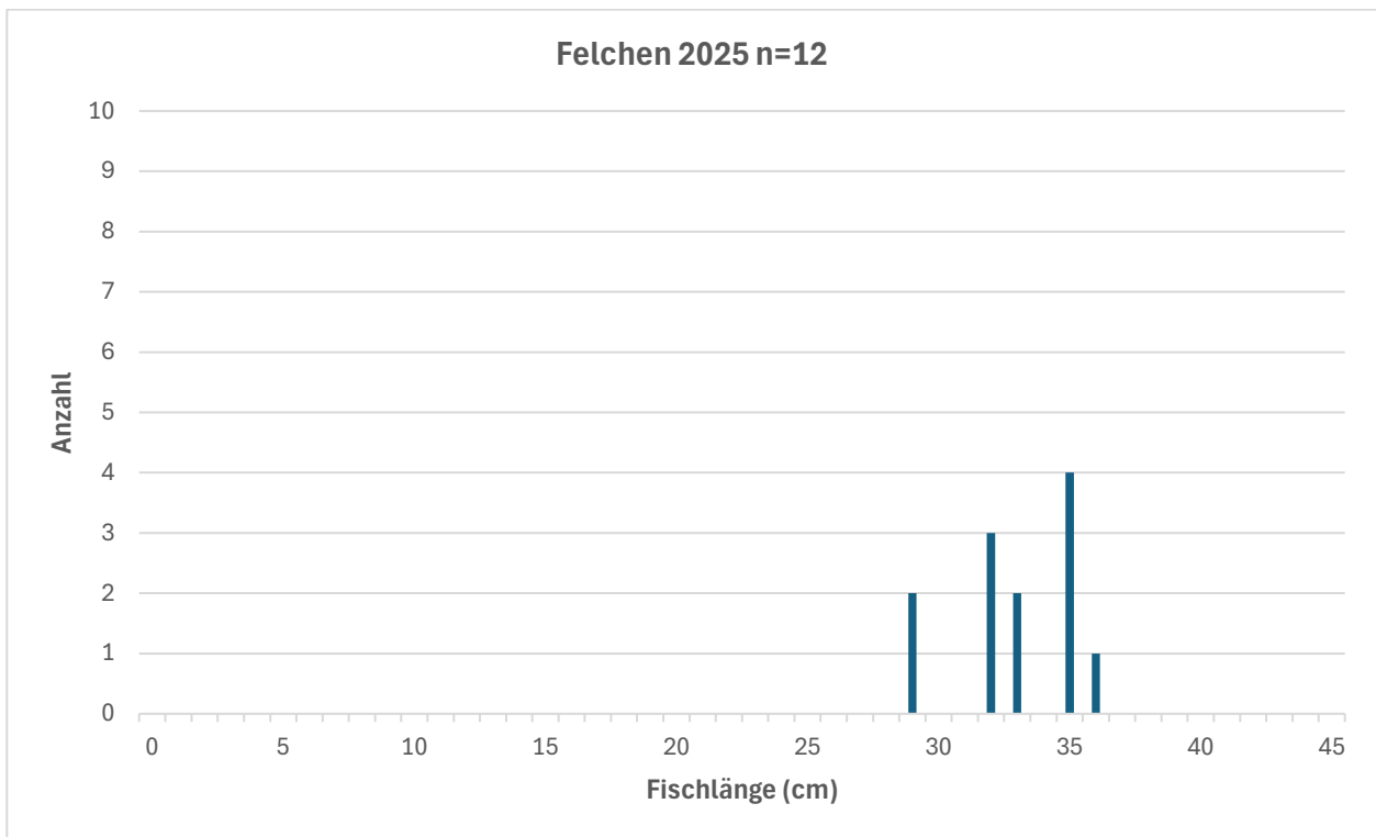
Abb. 77 Längen-Häufigkeitsverteilung Felchen/Renke - Alpenrhein (seit 2024 ganzjährig geschont).
