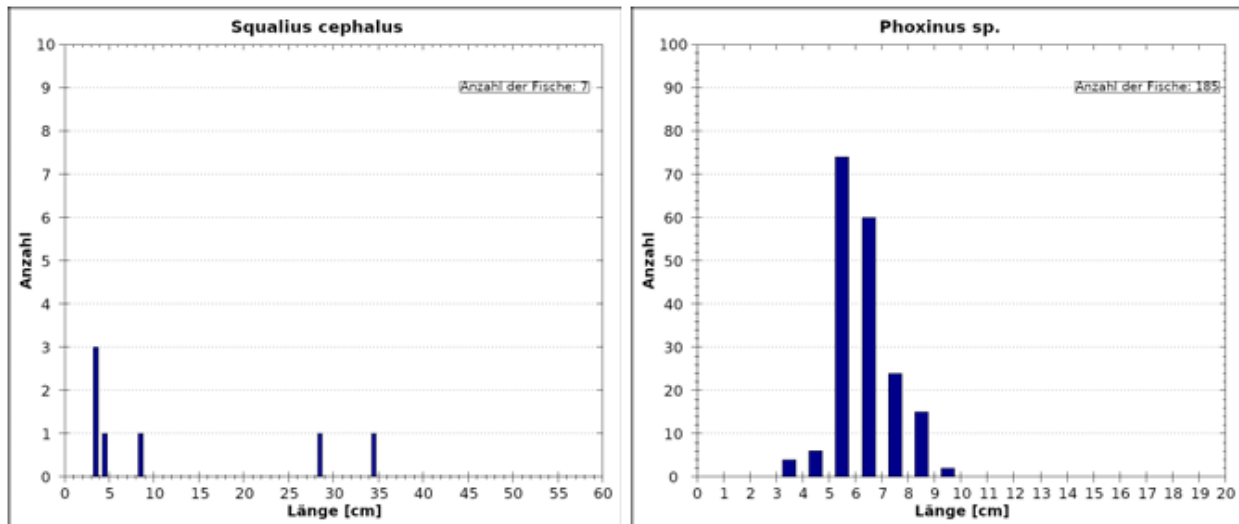
Abb. 99 Längenfrequenzdiagramm der typischen Begleitarten Aitel (links, Bewertung 4) und Elritze (rechts, Bewertung 1)
