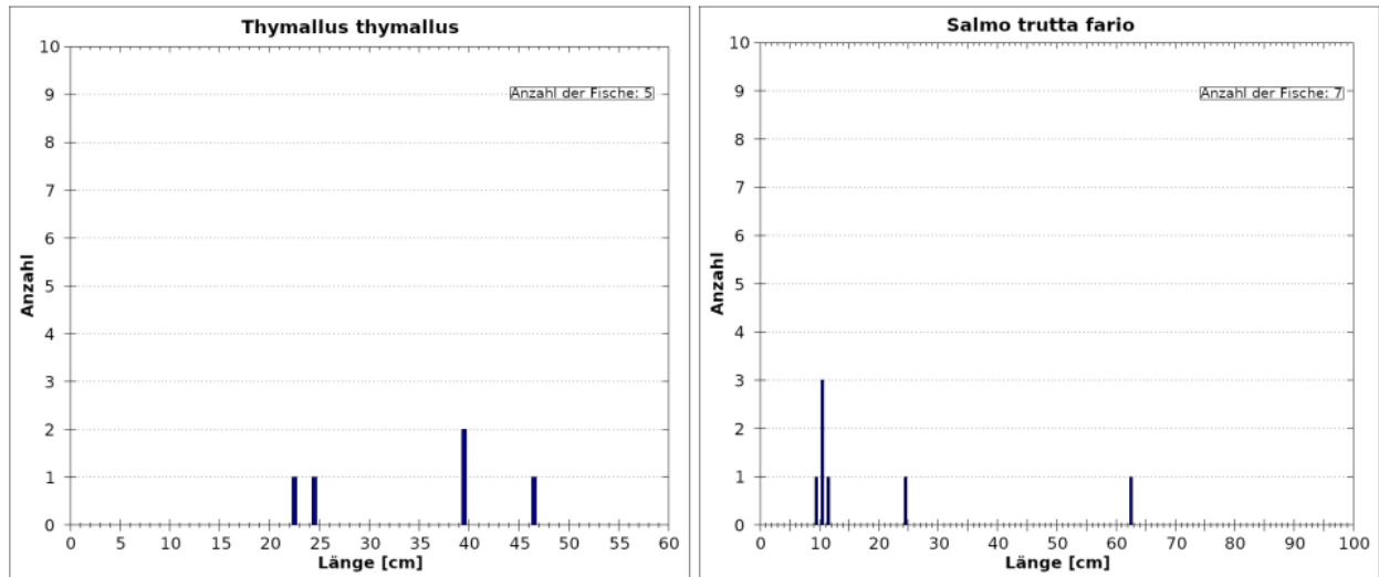
Abb. 40 Längenfrequenzdiagramm der Leitart Äsche (links) und Bachforelle (rechts) – RHE 4.
