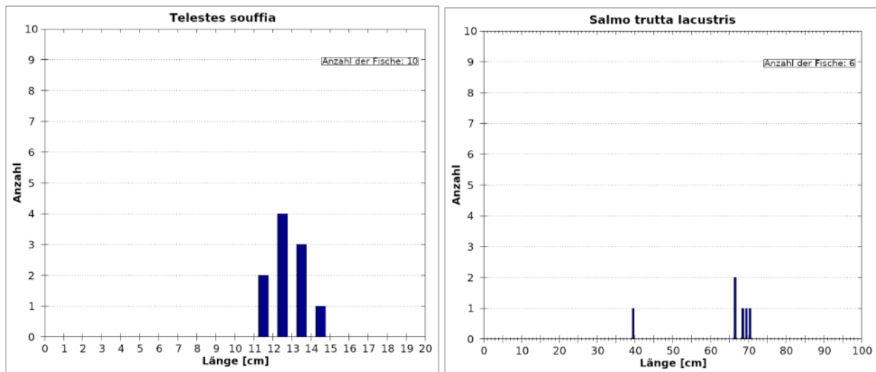
Abb. 25 Längenfrequenzdiagramm der Leitfischart Strömer (links), sowie der typischen Begleitfischart Seeforelle (rechts) – RHE 1.
