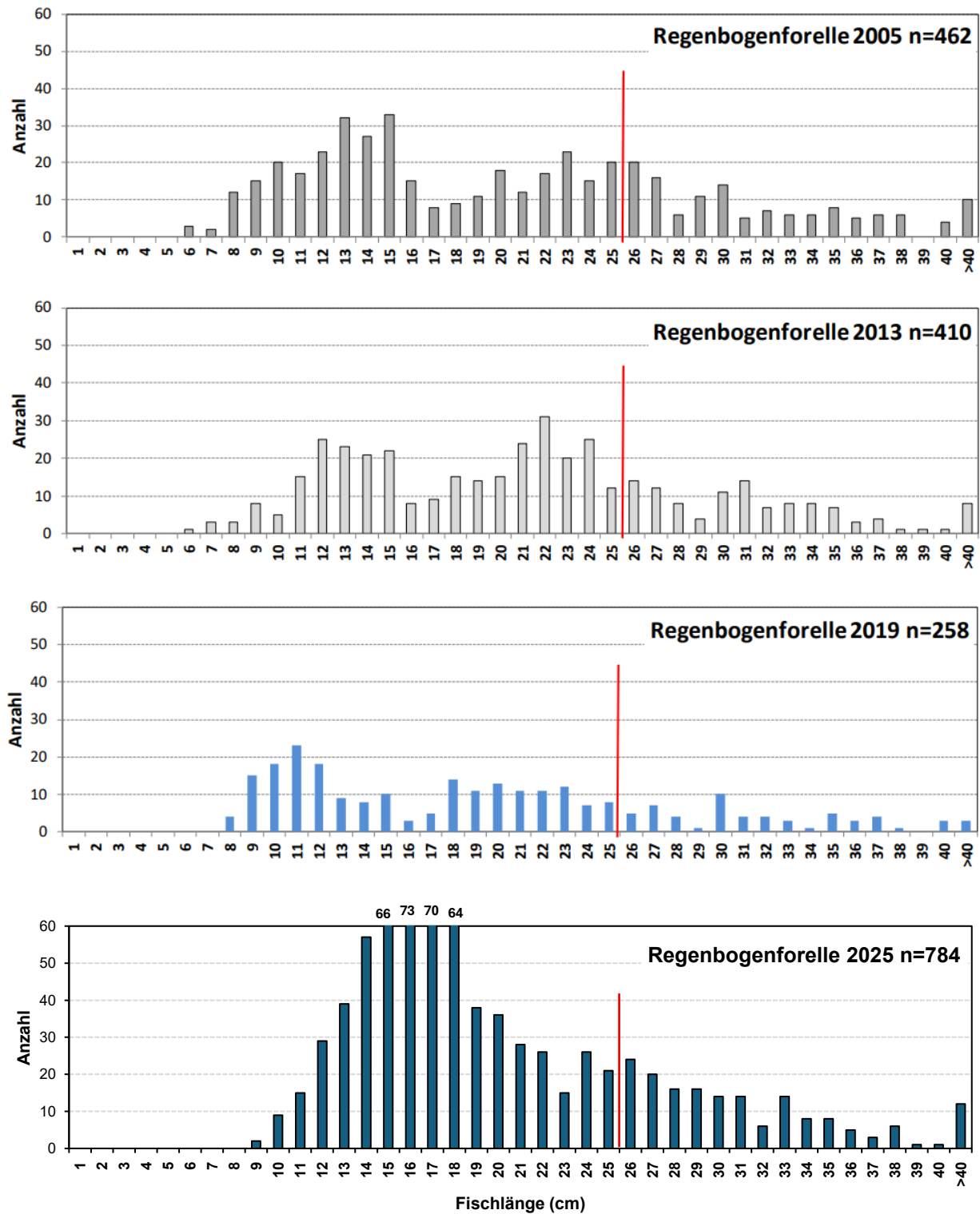
Abb. 83 Längen-Häufigkeitsverteilungen Regenbogenforelle – 2005, 2013, 2019 und 2025 – Alpenrhein.
