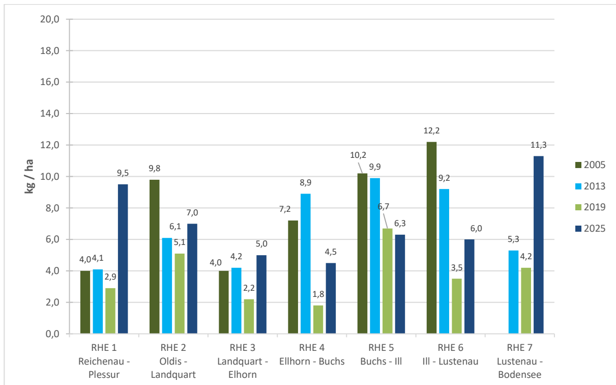
Abb. 81 Vergleich Biomasse pro Abschnitt 2005, 2013, 2019 und 2025 - Alpenrhein
