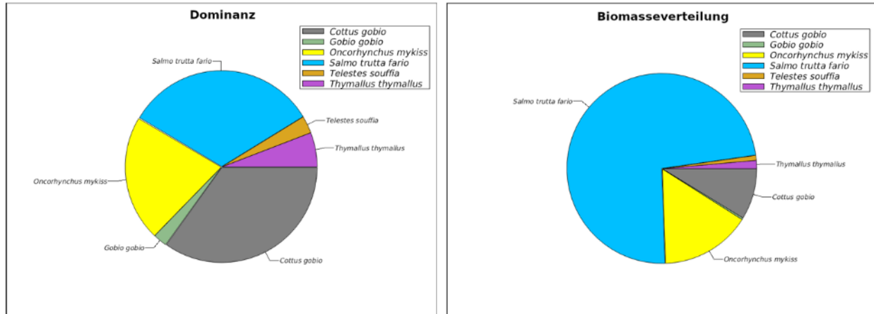
Abb. 105 Dominanz und Biomasserverteilung Ill – Feldkirch.
