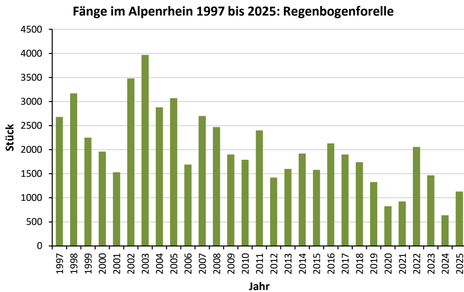
Abb. 114 Entwicklung Fangzahlen Regenbogenforelle 1997 bis 2025.
