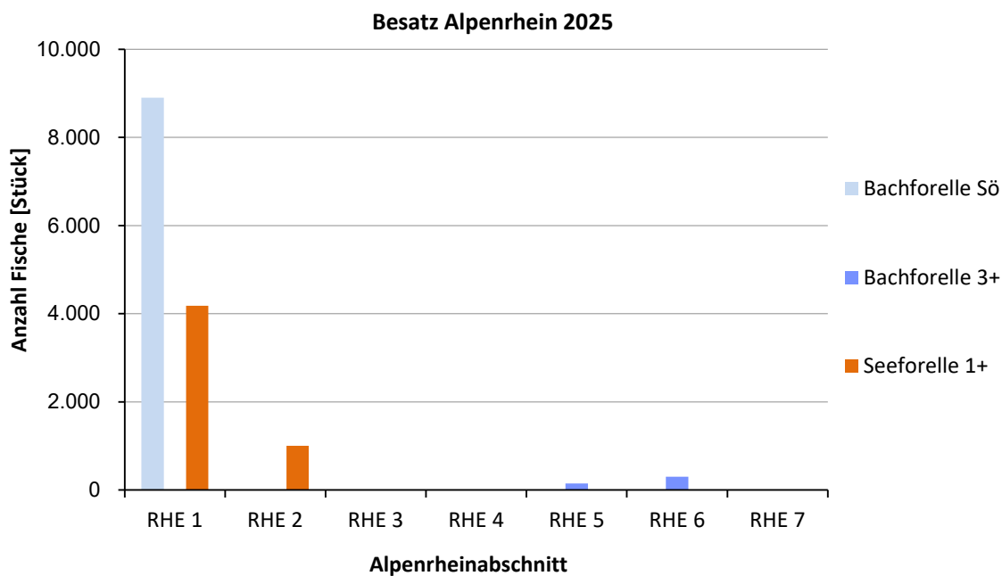
Abb. 116 Fischbesatz (Individuenzahlen), der 2025 direkt in den Alpenrhein erfolgte. Total: 14.530 Stück. Altersklassen: Sö = Sömmerlinge; 1+ = Einjährig; 3+ = 3-jährig (Hydra AG in prep).
