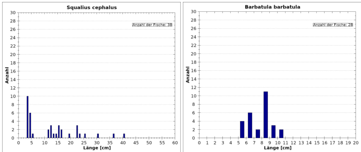
Abb. 61 Längenfrequenzdiagramm der typischen Begleitfischart Alet (links) und Bartgrundel (rechts) – RHE 7.
