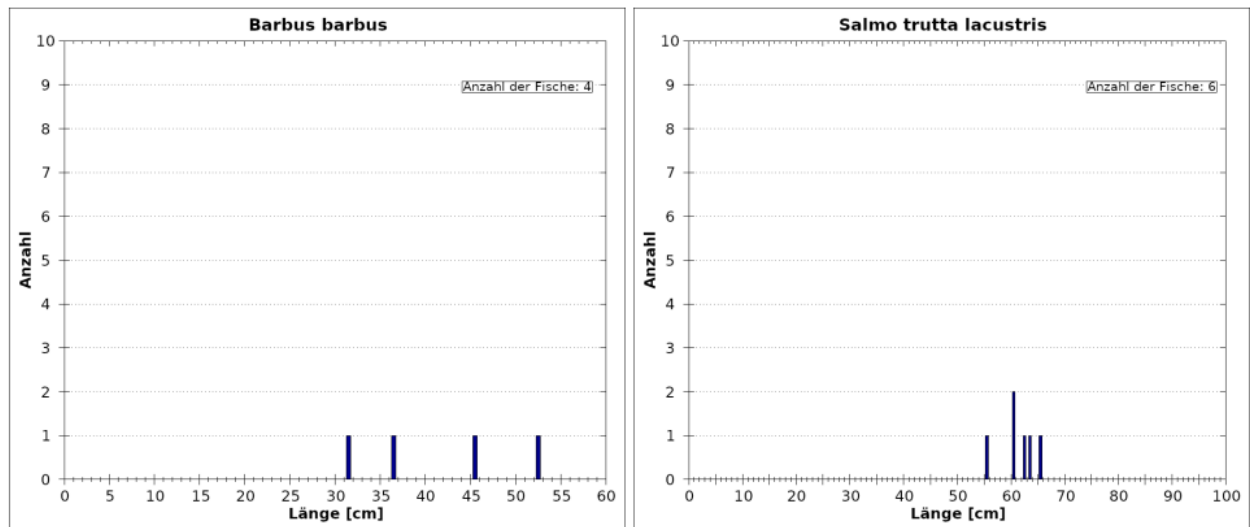
Abb. 62 Längenfrequenzdiagramm der typischen Begleitfischart Barbe (links) und Seeforelle (rechts) – RHE 7.
