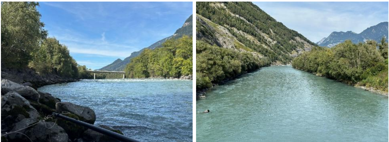
Abb. 21 Befischungsabschnitt RHE 1 – BR flussauf (links, © blattfisch e.U.) und flussab (rechts, © blattfisch e.U.).
