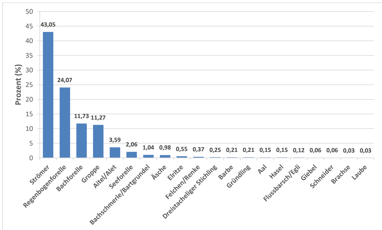
Abb. 63 Artenverteilung Alpenrhein 2025 – Gesamt.
