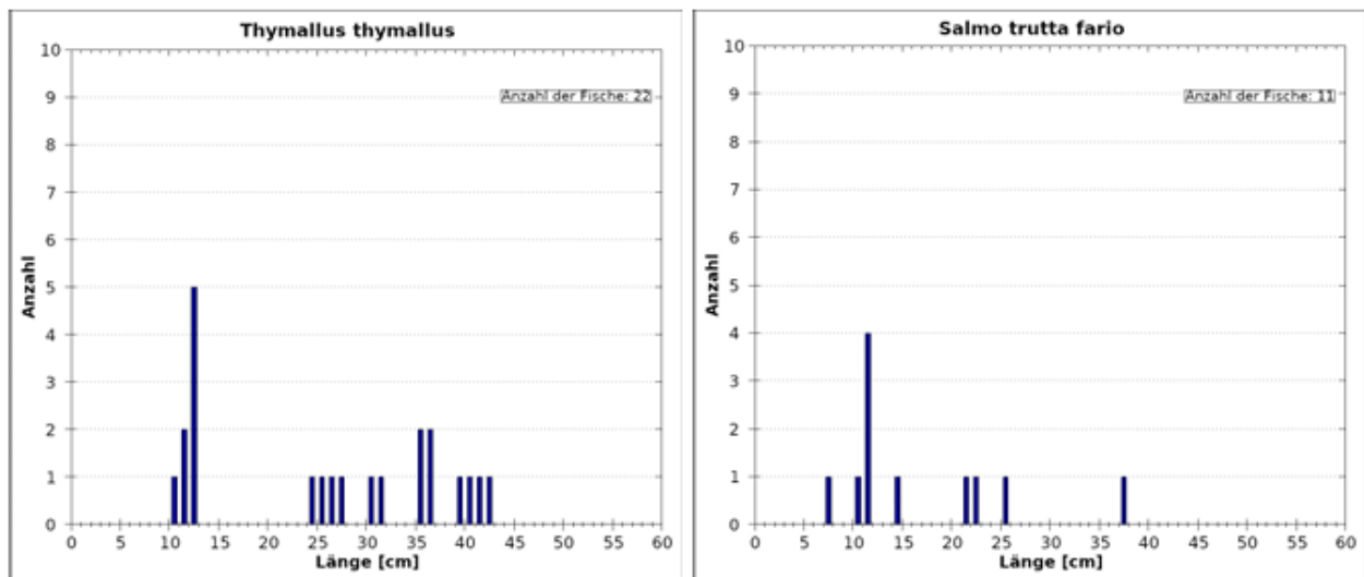
Abb. 102 Längenfrequenzdiagramm Äsche (links) und Bachforelle (rechts), jeweils mit Bewertung 3.
