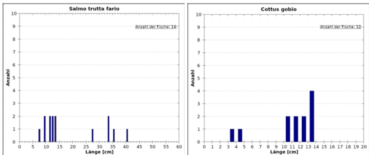
Abb. 106 Längefrequenzdiagramm Bachforelle (links) und Groppe (rechts), jeweils mit Bewertung 3.
