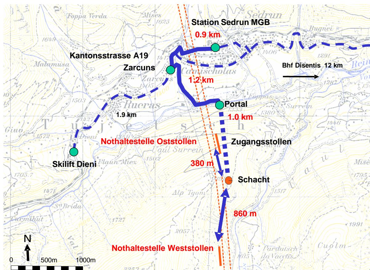
Abb. 2: Zugangsstollen Zwischenangriff Sedrun, Distanzen
