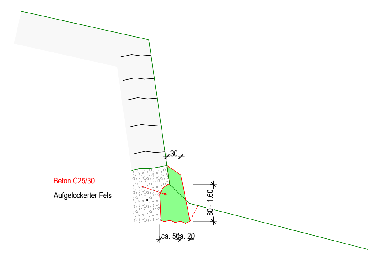
Unterfangung 1:50
