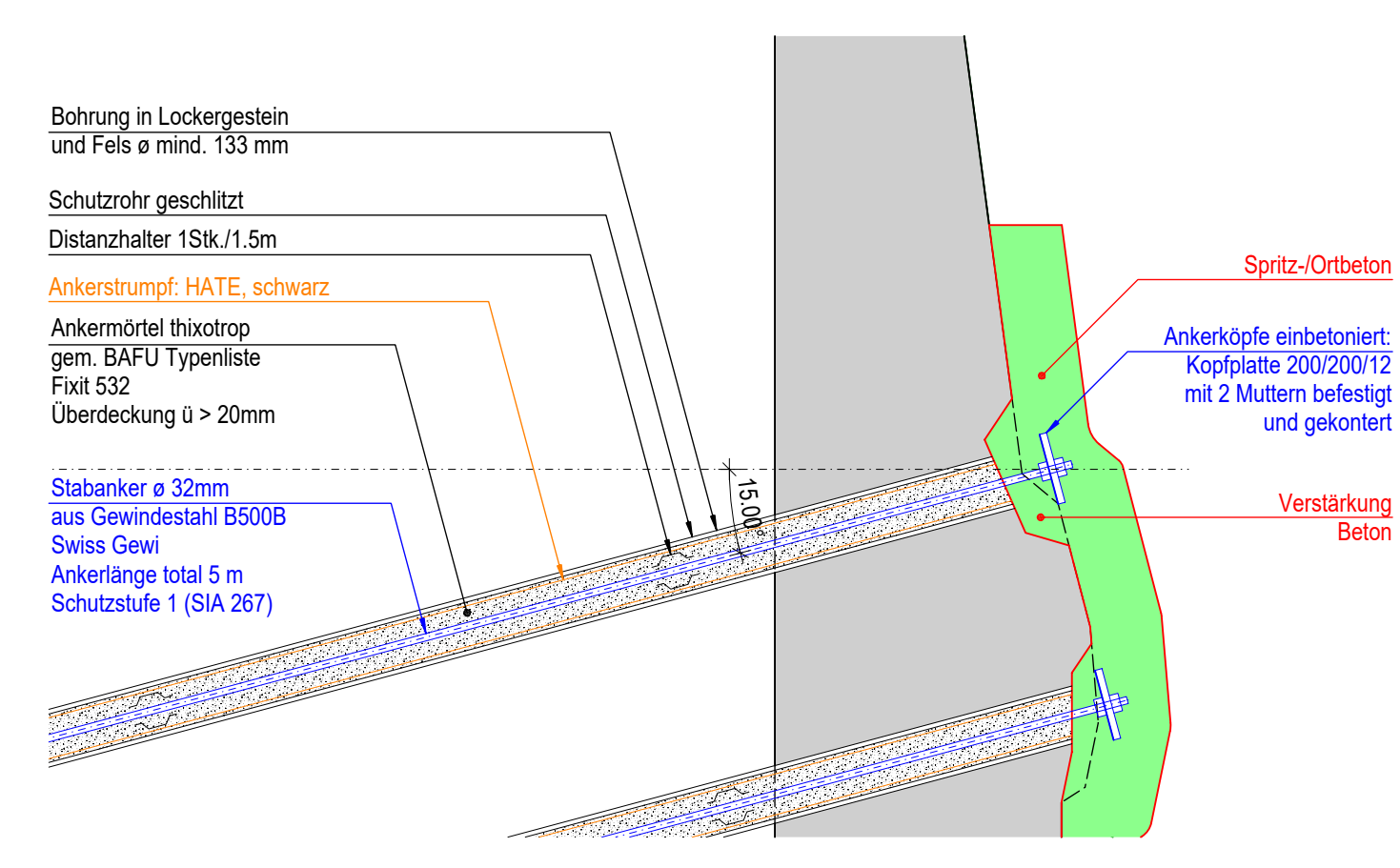
Anker zu Betonwand 1:20 Sperre 56
