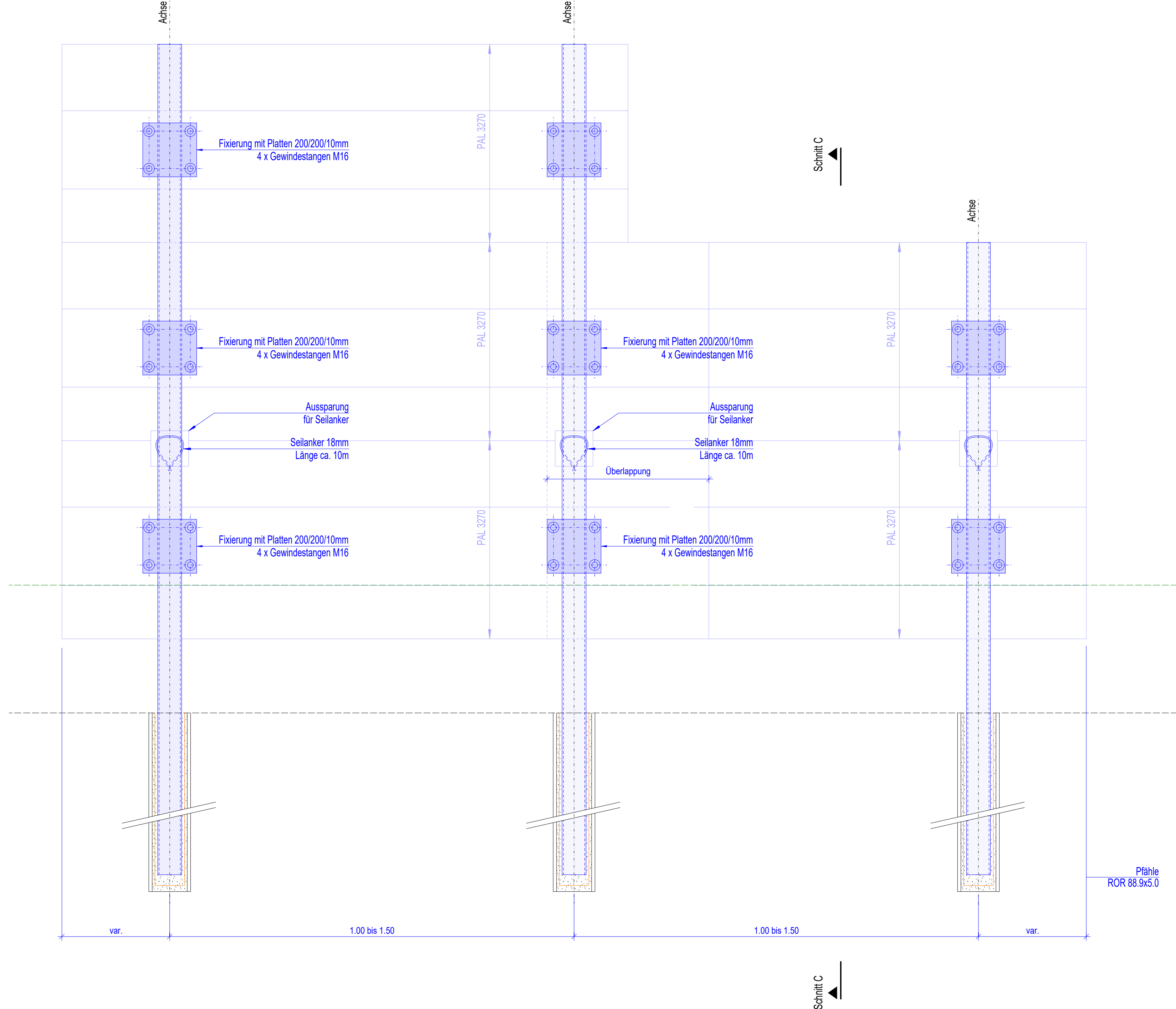
Seitlicher Erosionsschutz Ansicht D - D 1:10
