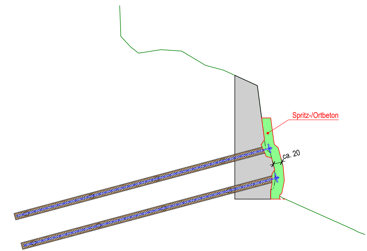
Betonwand 1:50 Sperre 56
