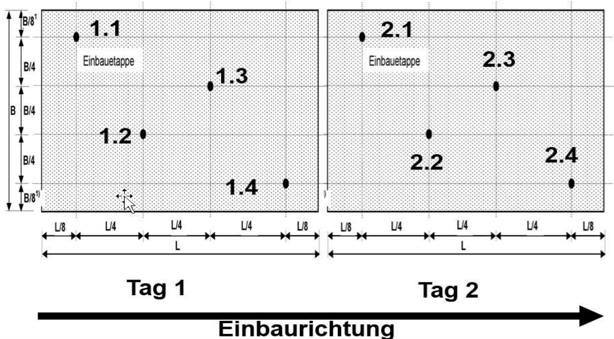
Abbildung: Entnahmeplan für Bohrkerne
