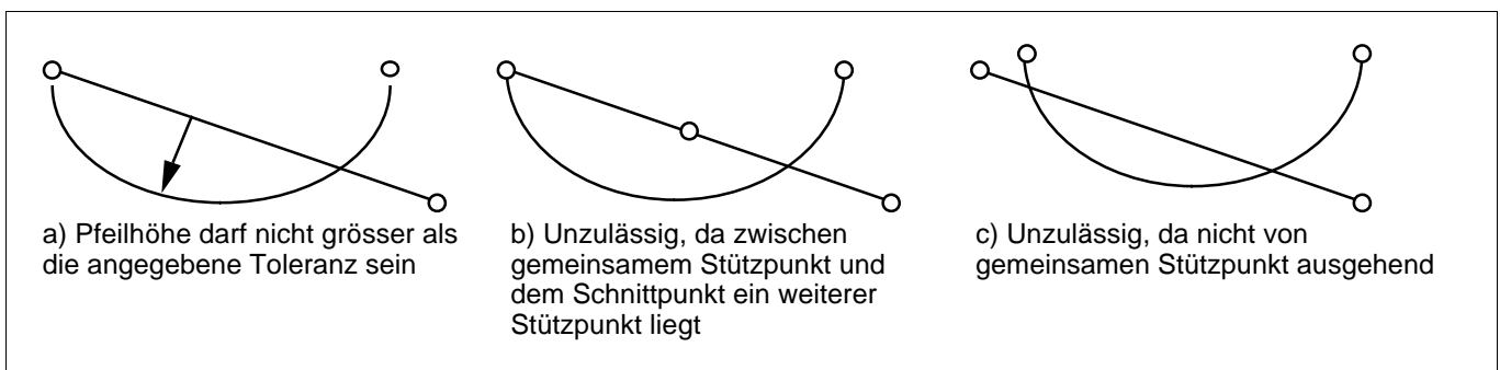
Abbildung 6: Toleranz (a) und unzulässige Überschneidungen (b+c) von Linienzügen
