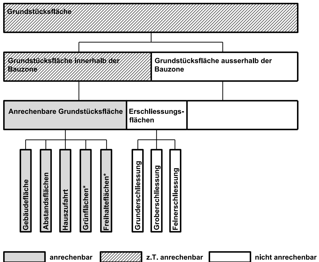
Figur 8.1 Anrechenbare Grundstücksfläche
