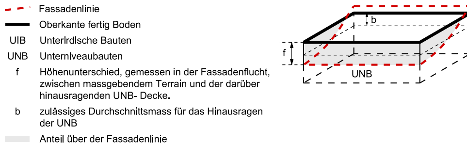
Figur 2.4 und 2.5 Unterirdische Bauten, Unterniveaubauten
