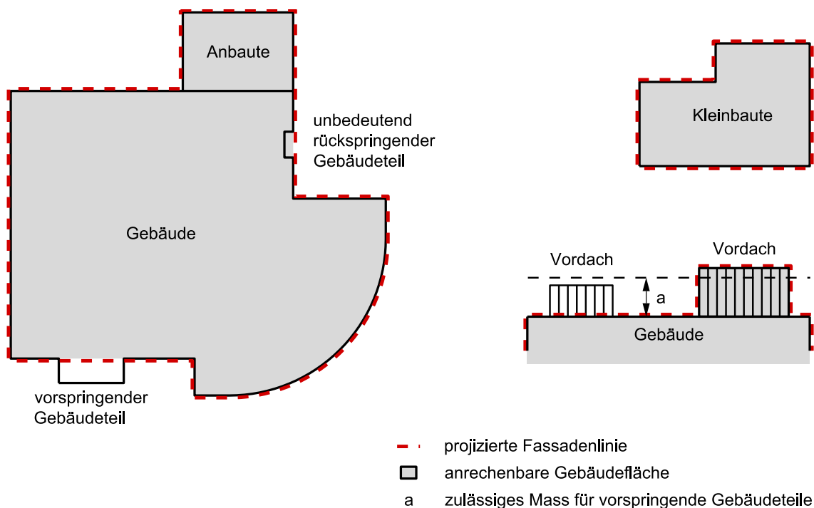
Figur 8.4 Anrechenbare Gebäudefläche
