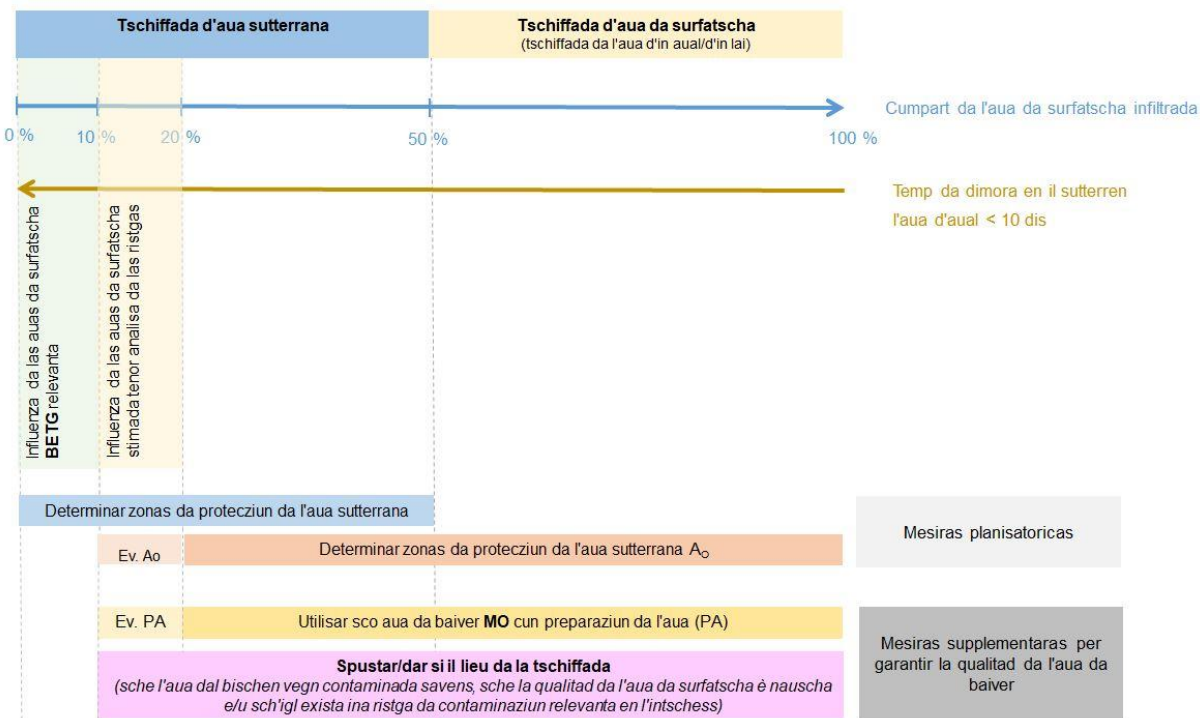
Illustraziun 2: Schema per giuditgar tschiffadas cun aua da surfatscha infiltrada
