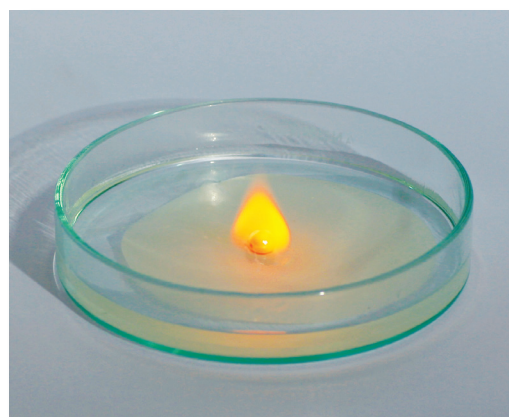
Foto: sodio in acqua, Thomas Seilnacht, Germania, www.seilnacht.com
