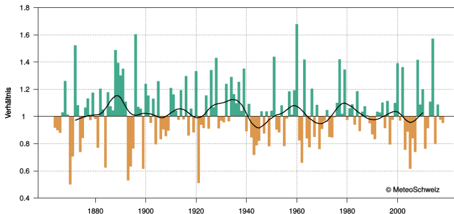
Abbildung 7. Jährliche Niederschlagssumme über die Jahre 1864 bis 2018. Dargestellt ist die Abweichung zur Norm von 1961 bis 1990 für die Südschweiz. Jahre mit Niederschlagssummen über dem Normwert sind grün eingezeichnet, Jahre darunter gelb. Das 20-jährige gleitende Mittel ist als schwarze Linie eingezeichnet. Quelle: MeteoSchweiz, 2019d.
