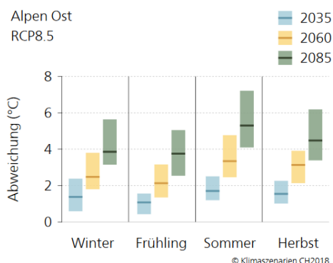
Abbildung 3. Erwartete Veränderung der Mitteltemperatur pro Saison für die Region Alpen Ost (RCP8.5). Quelle: CH2018-Webatlas.
