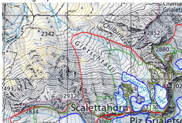
Abbildung 13. Die Ausdehnung des Scalettagletschers am Ende des Dischmatal in den Jahren 1920 (rot), 1970 (grün) und heute (blau). Quelle: Map.geo.admin.ch.
