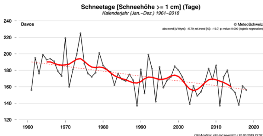
Abbildung 11. Entwicklung der jährlichen Anzahl Tage mit einer Schneedecke (mehr als 1 cm Schnee am Boden) über die Jahre 1961 bis 2018 in Davos. Das 20-jährige gleitende Mittel ist fett rot eingezeichnet, der lineare Trend ist rot gestrichelt dargestellt. Quelle: MeteoSchweiz, 2019b.
