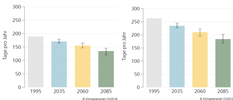
Abbildung 6. Erwartete Anzahl Frosttage pro Jahr in Davos (links) und auf Weissfluhjoch (rechts) unter dem Emissionsszenario RCP8.5. Quelle: CH2018-Webatlas.
