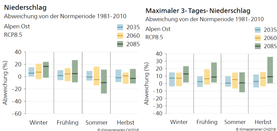
Abbildung 8. Erwartete Veränderungen der Niederschlagsmenge und der -intensität pro Saison unter dem Emissionsszenario RCP8.5 für die Region Alpen Ost. Quelle: CH2018-Webatlas.
