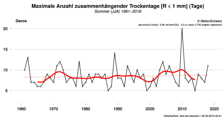
Abbildung 9. Maximale Anzahl zusammenhängender Trockentage in Davos im Sommer (Juni, Juli, August; Regensmengen weniger als 1mm) über die Jahre 1961 bis 2018. Quelle: MeteoSchweiz, 2019b.
