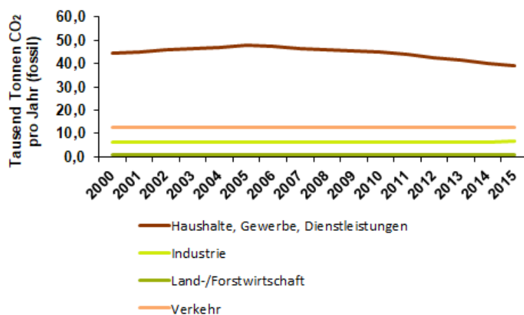
Abbildung 1. Emissionen an fossilem CO 2 in Davos. Quelle: Emissionskataster.
