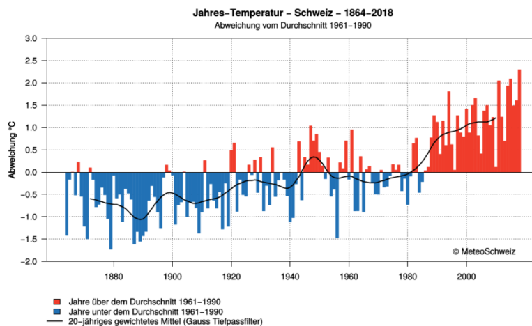
Abbildung 2. Jahres-Mitteltemperatur der Schweiz über die Jahre 1864 bis 2018. Dargestellt sind die jährlichen Abweichungen im Durchschnitt der Jahre 1961 bis 1990.
