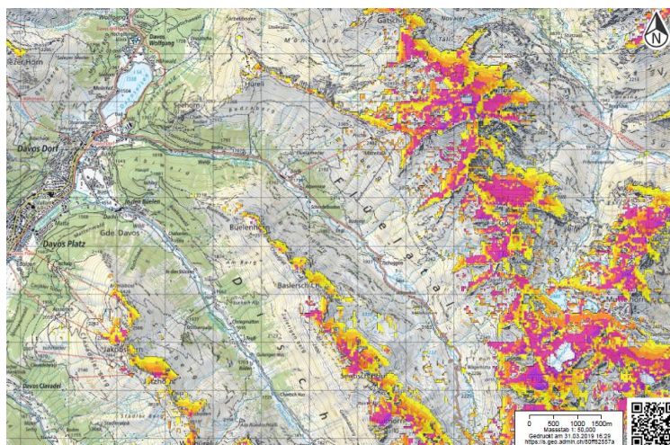
Abbildung 14. Permafrosthinweiskarte für Davos. Quelle: map.geo.admin.ch/Permafrosthinweiskarte .
