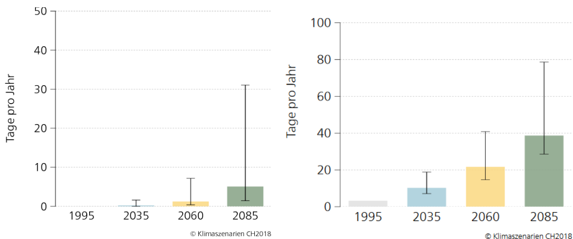
Abbildung 4. Links: Entwicklung der Anzahl Hitzetage ( T_{\max} \geq 30\text{ °C} ) in Davos bis gegen Ende des 21. Jahrhunderts unter dem Szenario RCP8.5. Rechts: Erwartete Entwicklung der Anzahl Sommertage ( T_{\max} \geq 25\text{ °C} ) in Davos. Quelle: CH2018-Webatlas.
