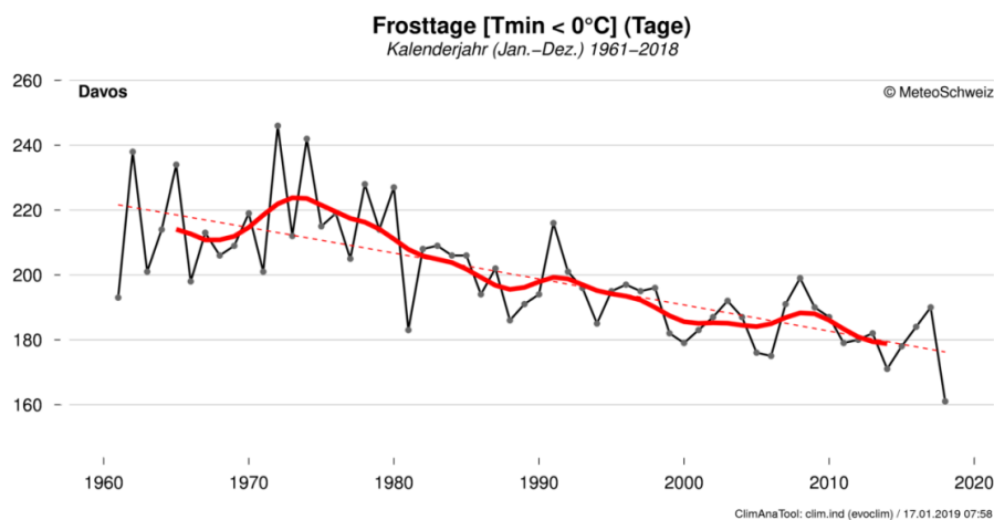
Abbildung 5. Ein Frosttag ist ein Tag mit einer Minimumtemperatur von unter null Grad. Die Frosttage haben in den vergangenen Jahren in Davos deutlich abgenommen. Quelle: MeteoSchweiz, 2019b.
