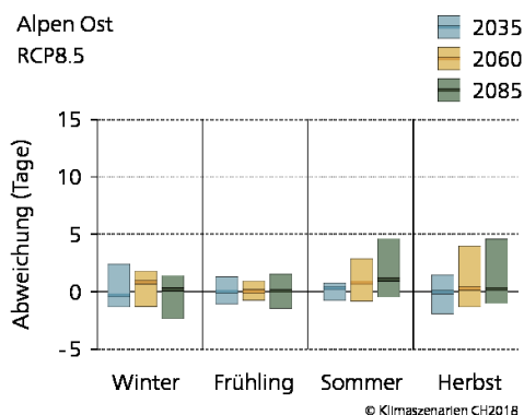
Abbildung 10. Abweichung der maximalen Anzahl zusammenhängender Trockentage pro Saison unter dem Emissionsszenario RCP8.5 für die Regionen Alpen Ost. Quelle: CH2018-Webatlas.
