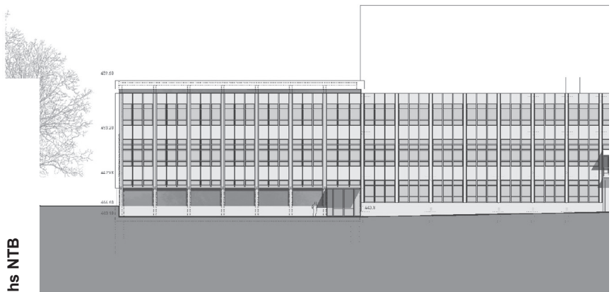
Ansicht Süd
