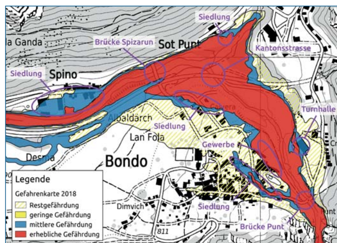
Bild 9. Gefahrenkarte Wasser 2017/18, basierend auf den seit den Ereignissen 2017 neu definierten Szenarien (Quelle: [4]).
