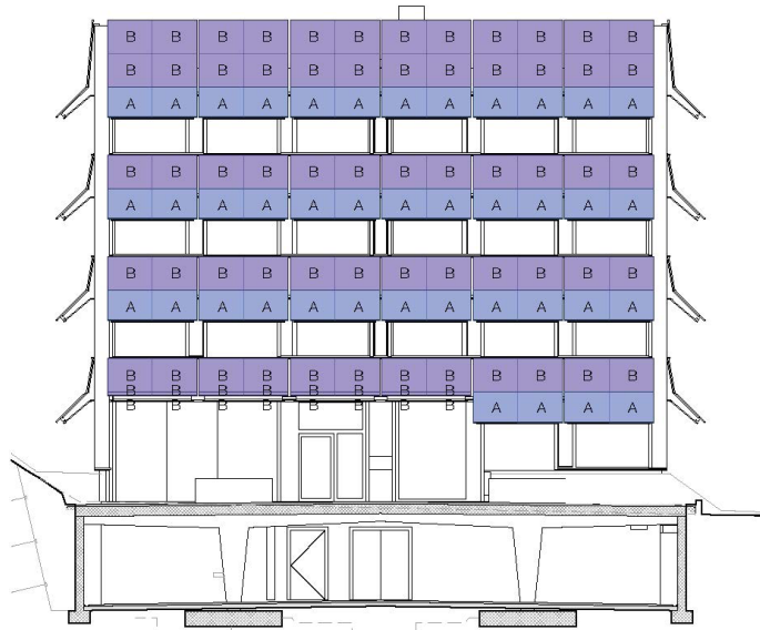
Photovoltaik-Module an der Fassade
