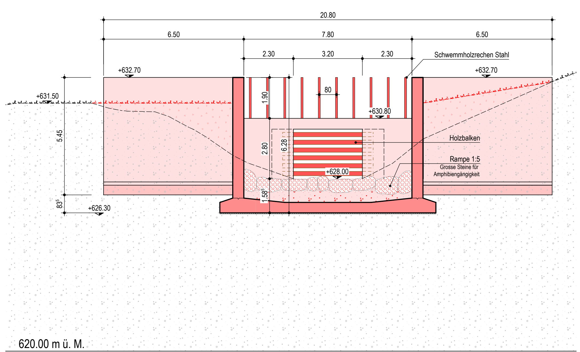
SCHNITT B-B 1:100 Querschnitt
