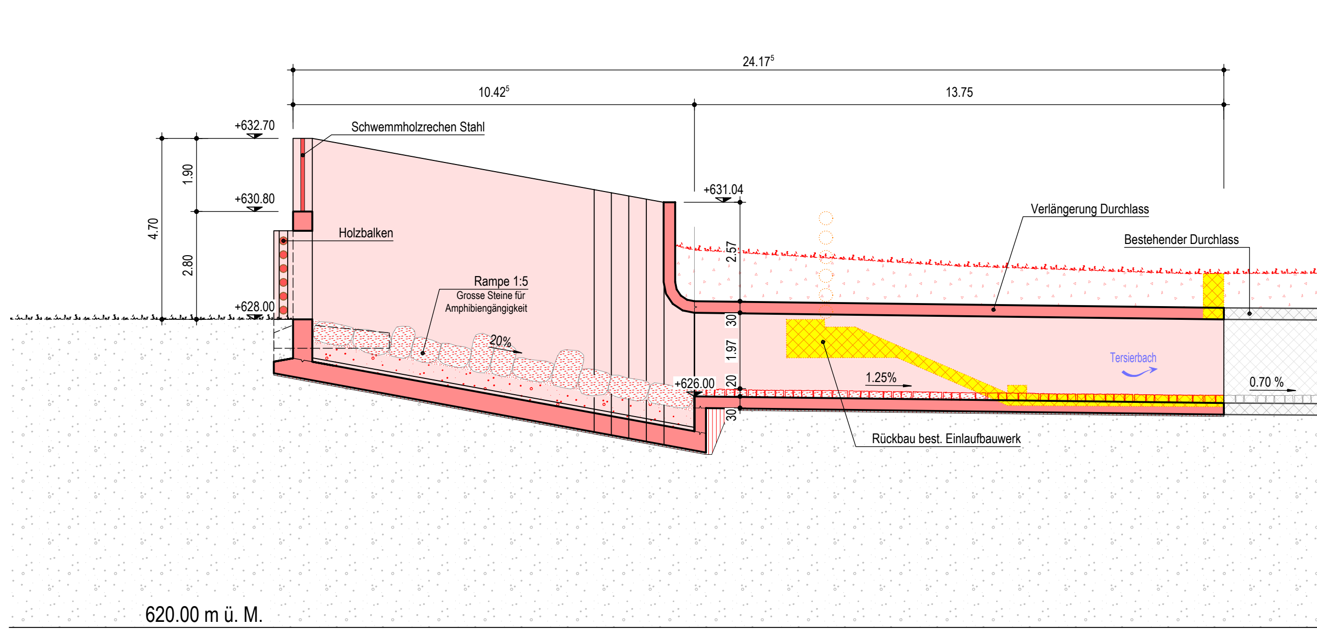
SCHNITT A-A 1:100 Längsschnitt
