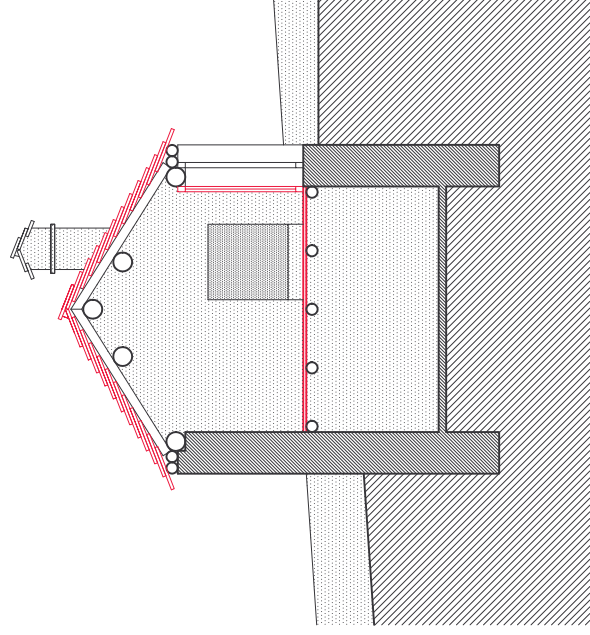
SEZIONE TRASVERSALE A-A
