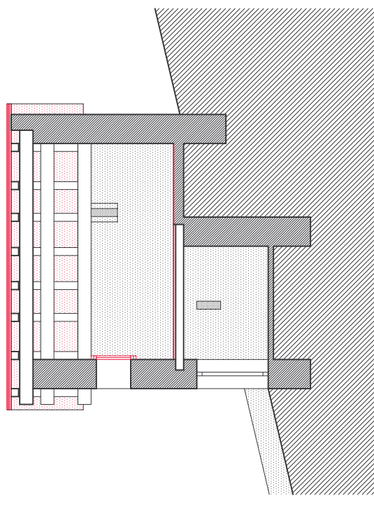
SEZIONE LONGITUDINALE B-B
