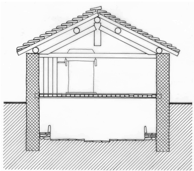
SEZIONE TRASVERSALE
