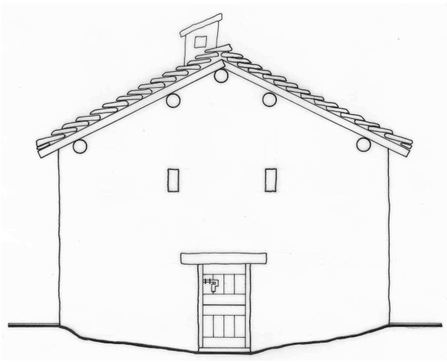
VISTA OVEST
