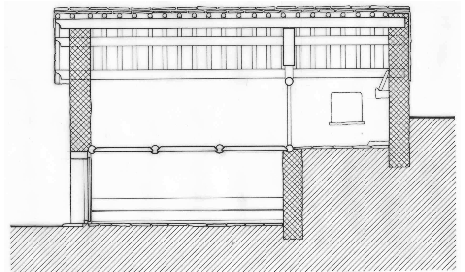
SEZIONE LONGITUDINALE
