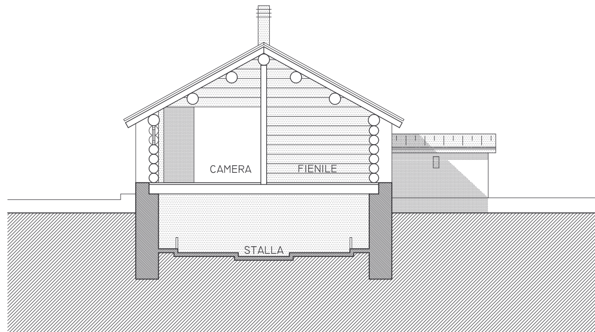
SEZIONE TRASVERSALE 1:100
