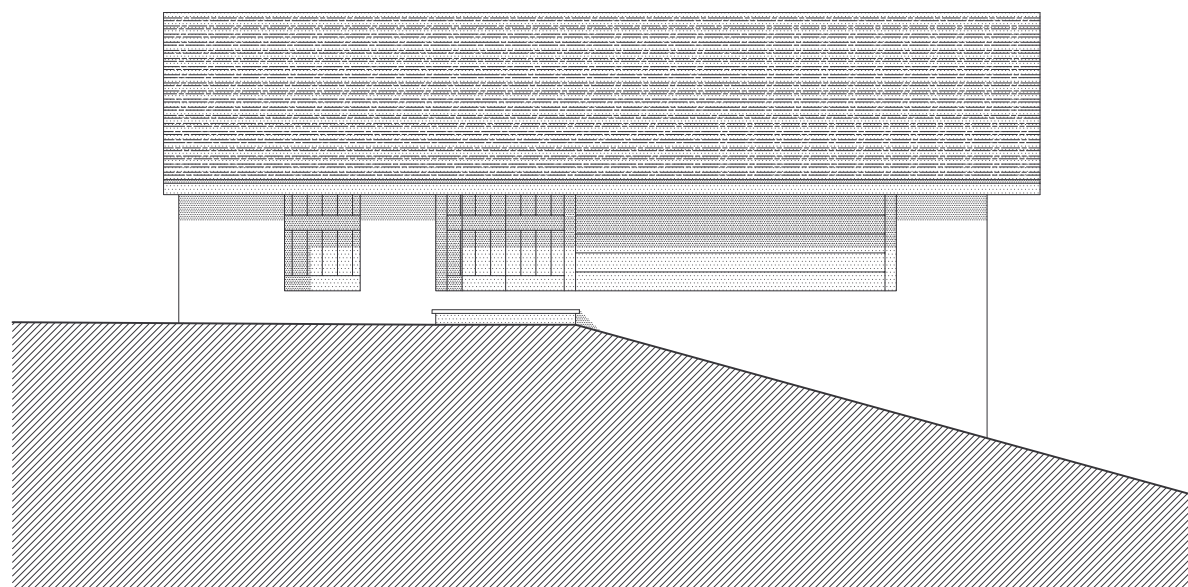
VISTA SUD-EST 1:100
