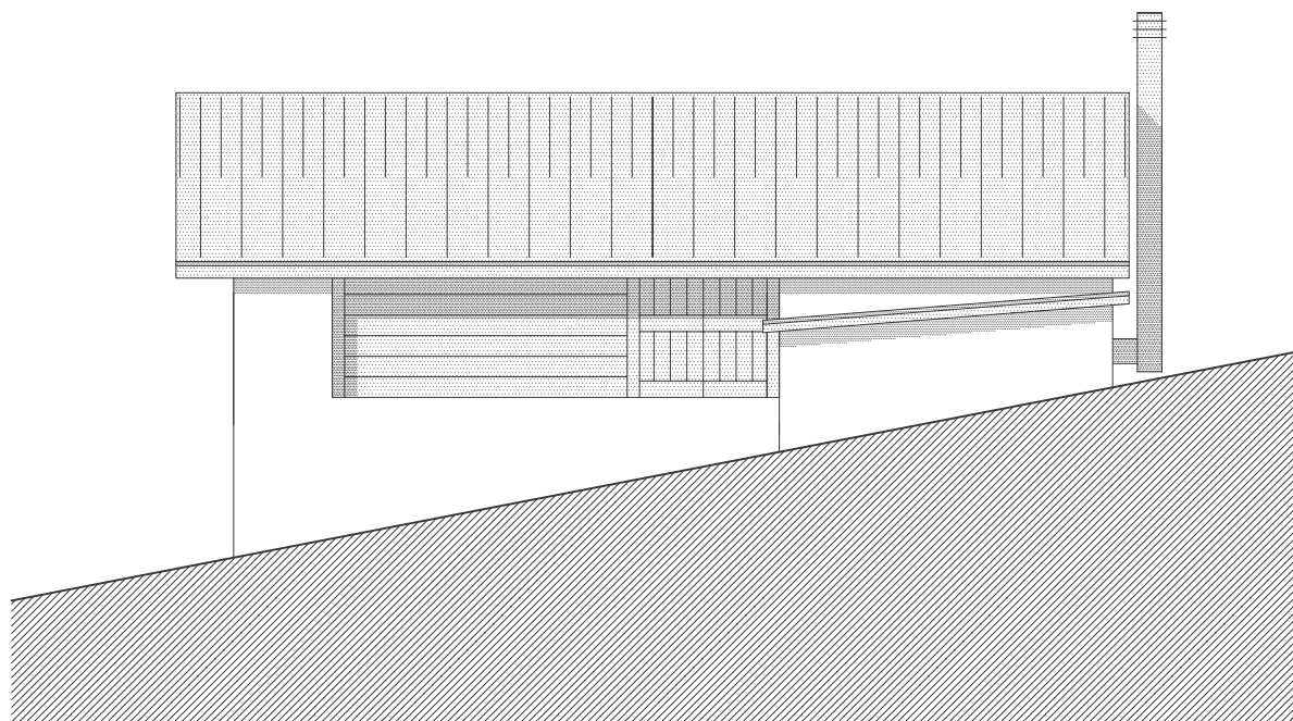
VISTA NORD-OVEST 1:100
