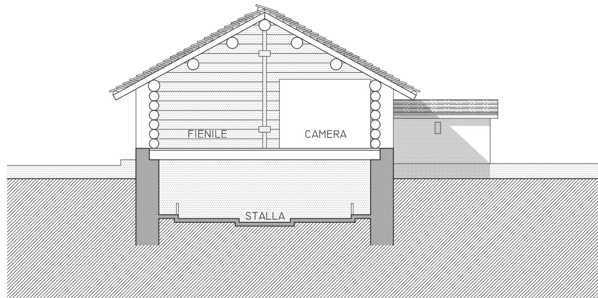
SEZIONE TRASVERSALE 1:100
