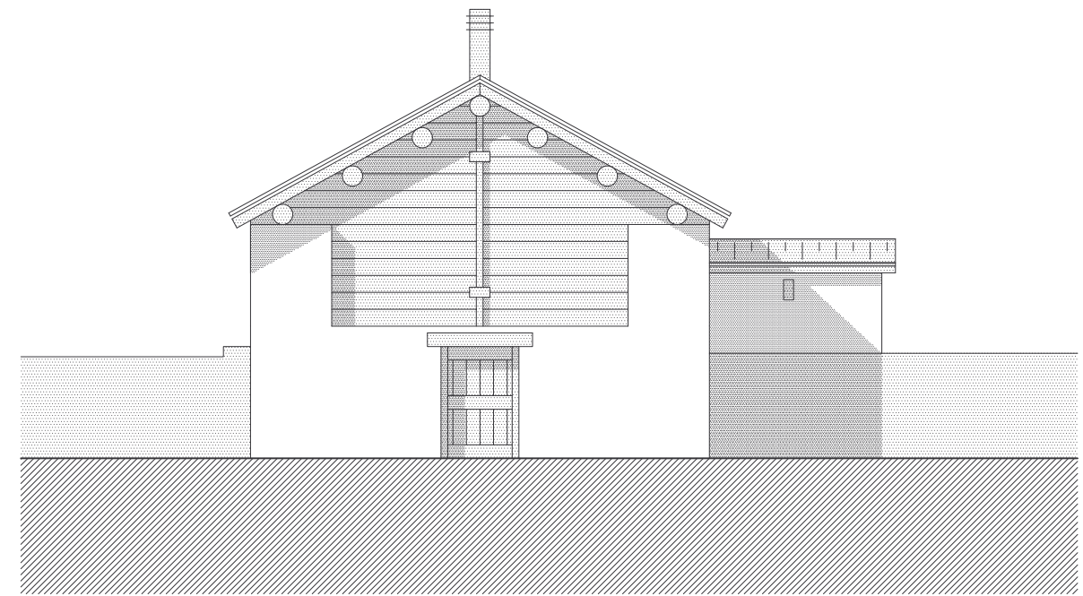
VISTA NORD-EST 1:100
