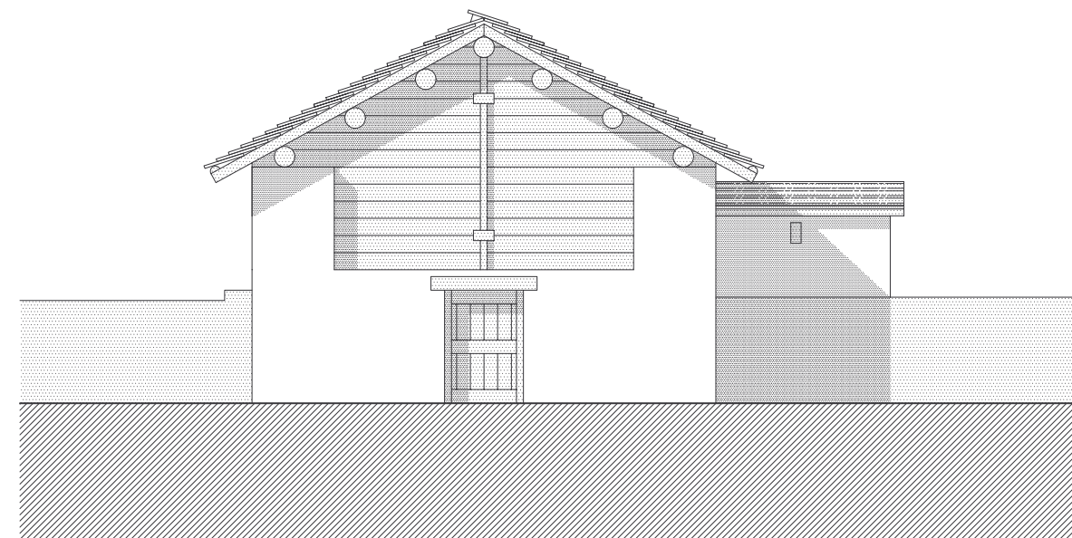
VISTA NORD-EST 1:100
